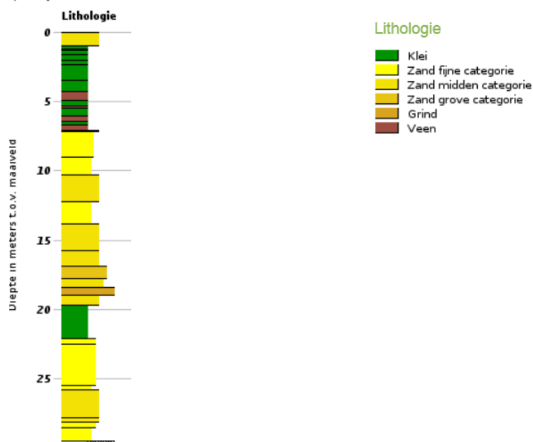
Afbeelding 2.1: Boorprofiel boring B20G0075
