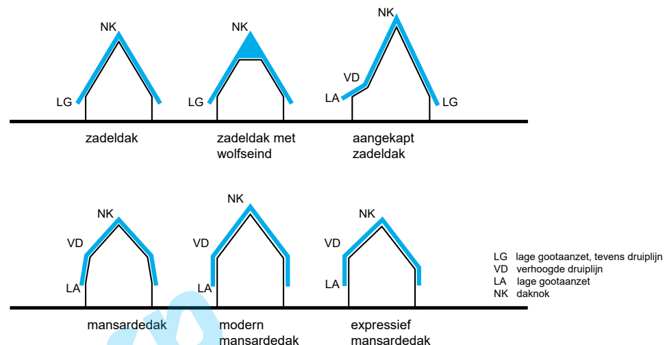
Mogelijke kapvormen in Klein Nooten
