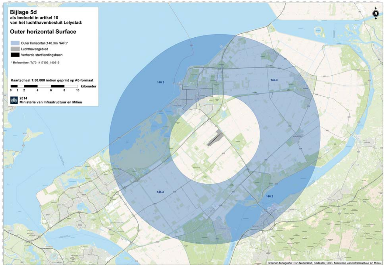
Kaart (1:50.000) met hoogtebeperkingen: Outer horizontal Surface
