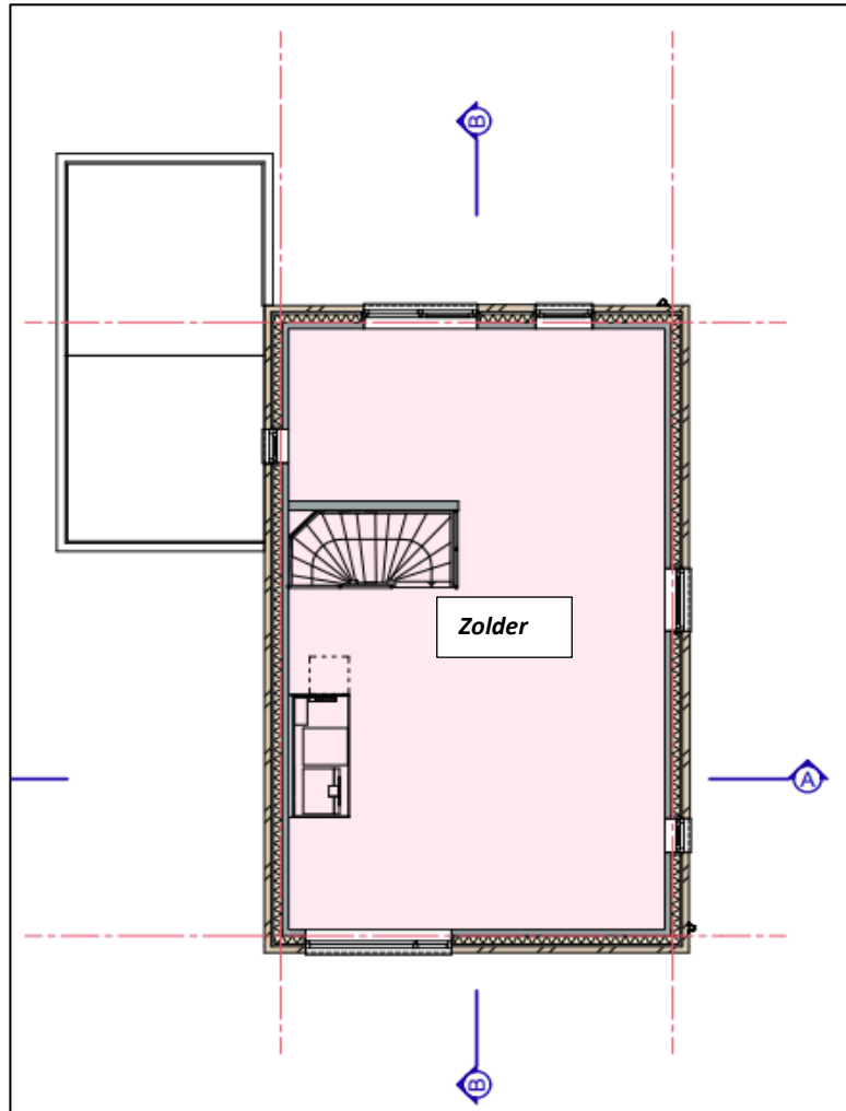
Plattegrond tweede verdieping stadswoningen (bron: Architectenburo Snijders en van Stekelenburg)
