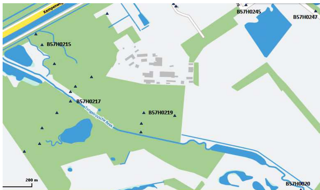
Figuur 2.3. Peilbuizen in het gebied. De geselecteerde peilbuizen (codenummer vermeld) hebben een diep filter dat de grondwaterstijghoogten in het watervoerende pakket weergeeft.
