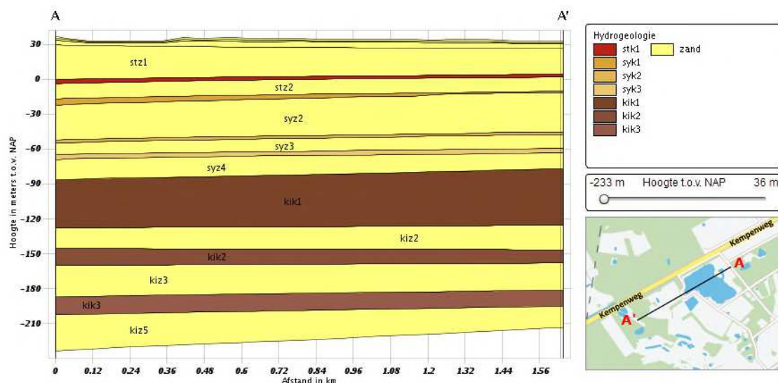
Figuur 2.1. Opbouw van de ondergrond volgens Regis II, versie 2.1. Met stz is Sterkel aangegeven. Boven Sterkel ligt nog de Formatie van Bortel. In het dwarsprofiel ligt de onderkant van Bortel op ca. NAP +30 m. De gele lagen zijn zand. De lagen met een bruine of rode kleur zijn (soms dunne) slechter doorlatende lagen.
