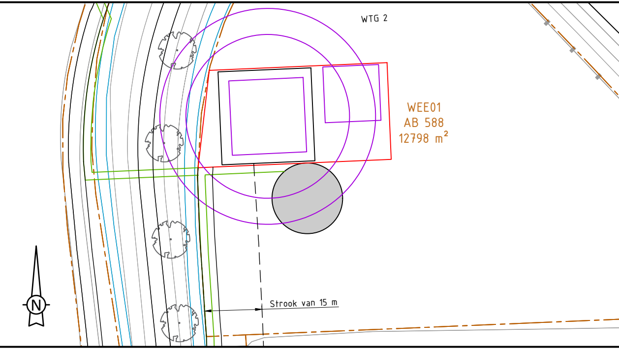
Overzicht WTG 3 - schaal 1:100
