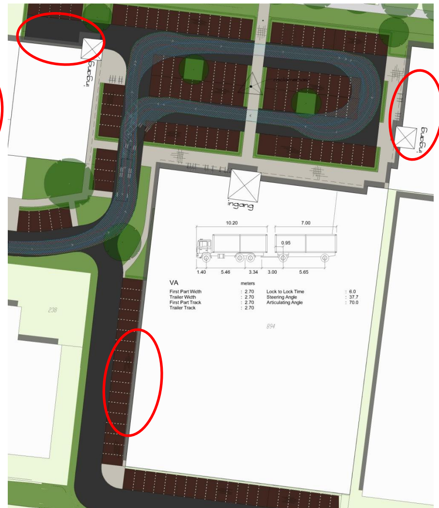
Figuur 15: rijcurves vrachtwagen met aanhanger
