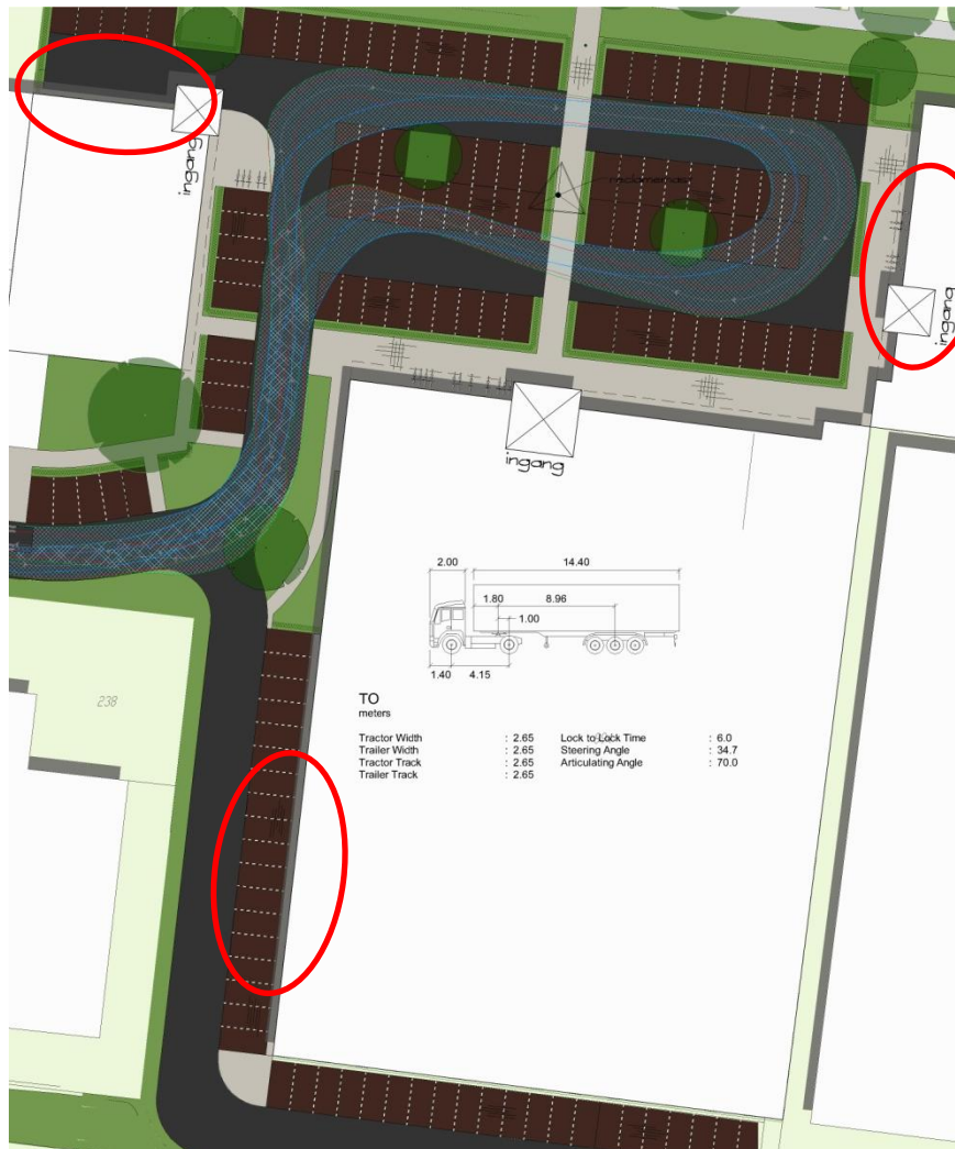
Figuur 17: rijcurves trekker met oplegger
