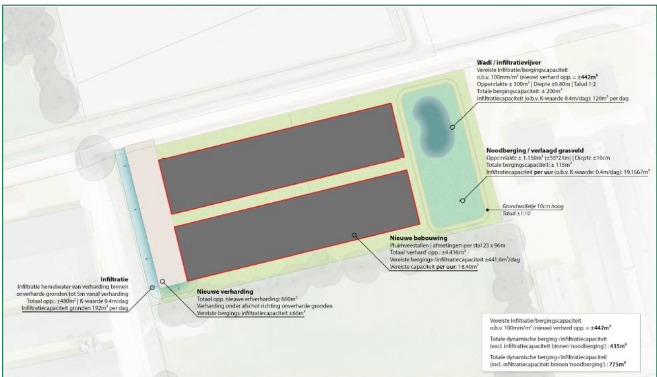
Figuur 8: Overzicht waterhuishouding planvoornemen
