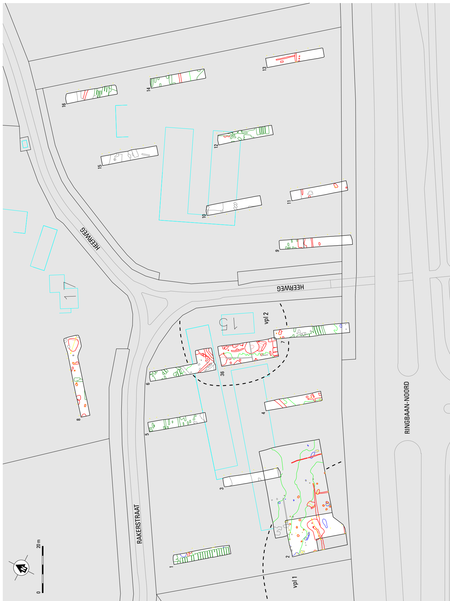
Fig. 3. Weert-Kampershoe Noord fase 3. Overzicht van de proefsleuven en sporen in deelgebied 2011-a (reeds aangelegde werkput niet wit opgevuld). Schaal 1:1000. rood grondsporen; groen bodemlagen; blauw natuurlijke sporen; donkergroen subrecent; grijs recent.
