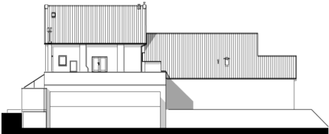
Achtergevel Schoolstraat 3 bestaande situatie | bron: Architectenzaak
