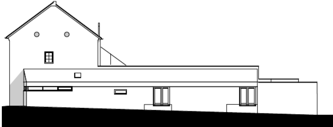
Rechter zijgevel Schoolstraat 3 bestaande situatie | bron: Architectenzaak
