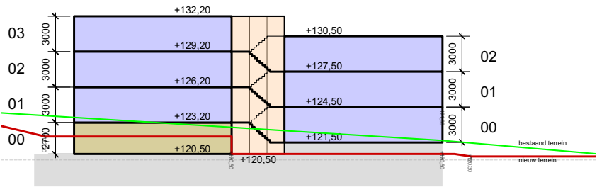
doorsnede 01 bestaand terrein afgegraven maakt dat de ZO-gevel iets is opgetild i.v.m. parkeren
