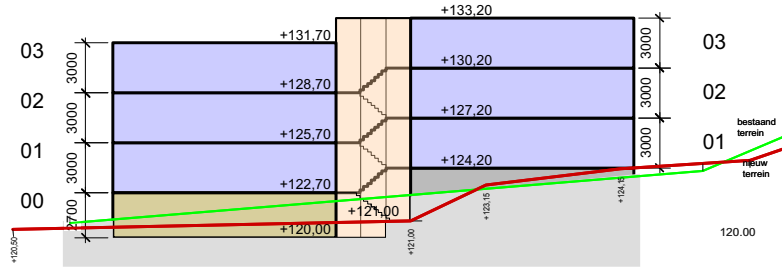
doorsnede 02
