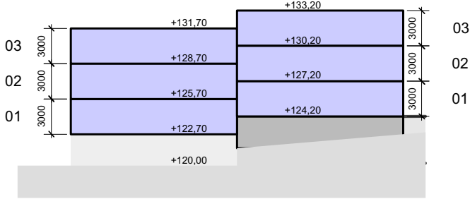
doorsnede 01
