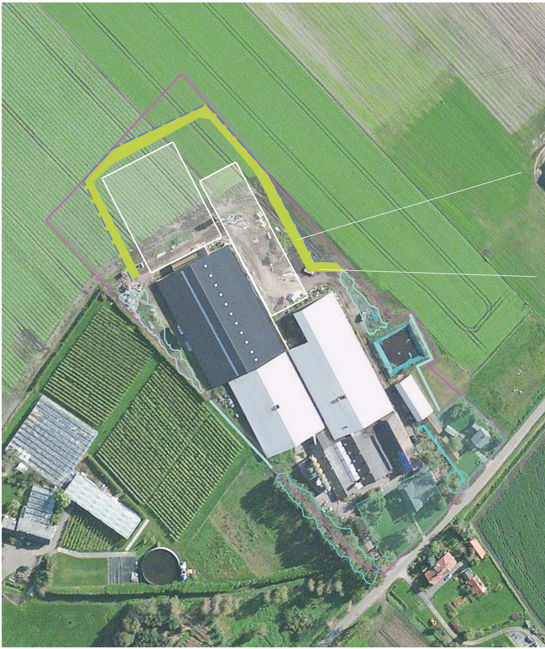
infiltratiesloot
