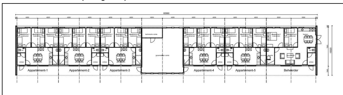
Figuur 2. Plantekening toekomstige situatie van het te realiseren woongebouw.
