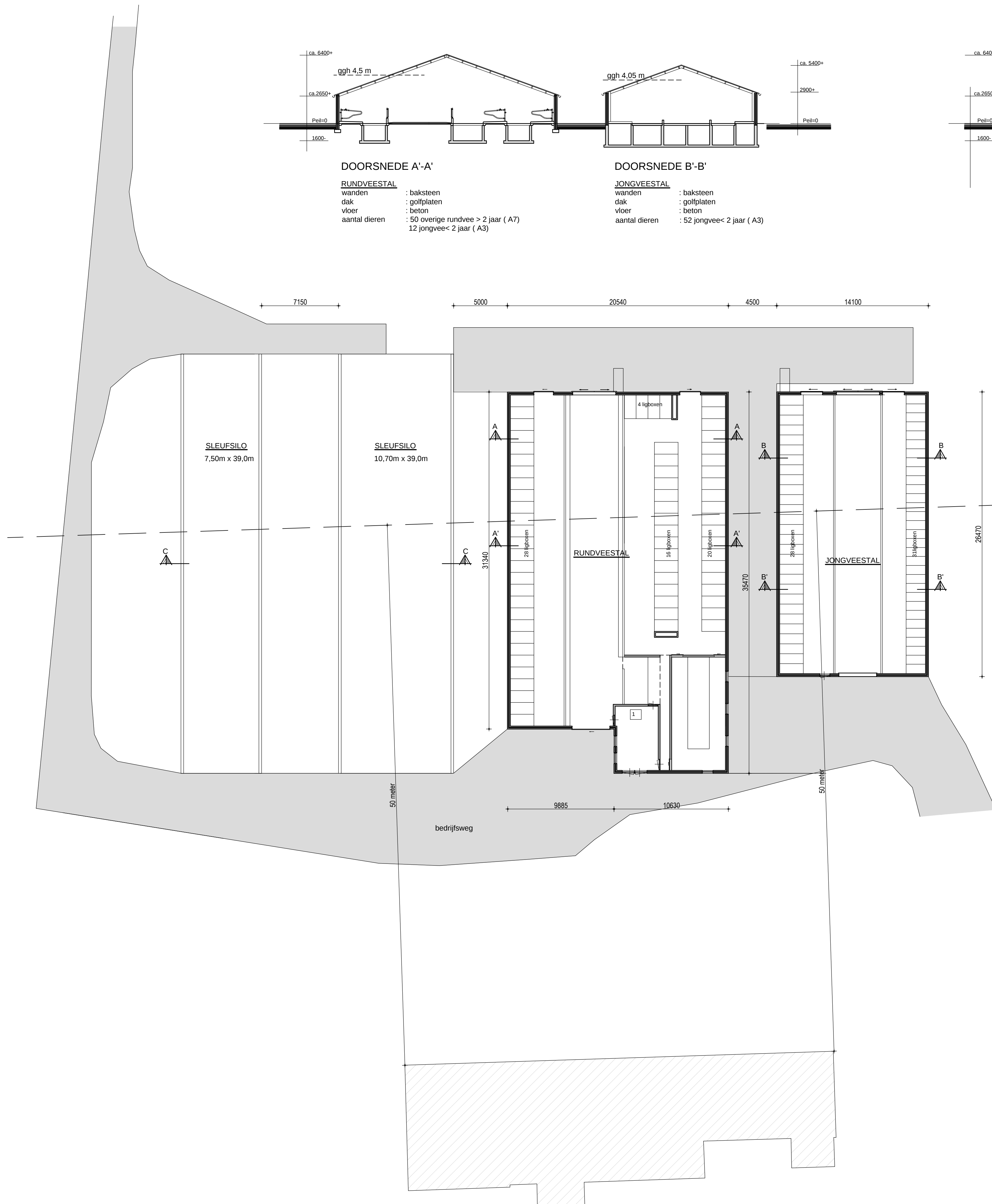
DOORSNEDE A-A
