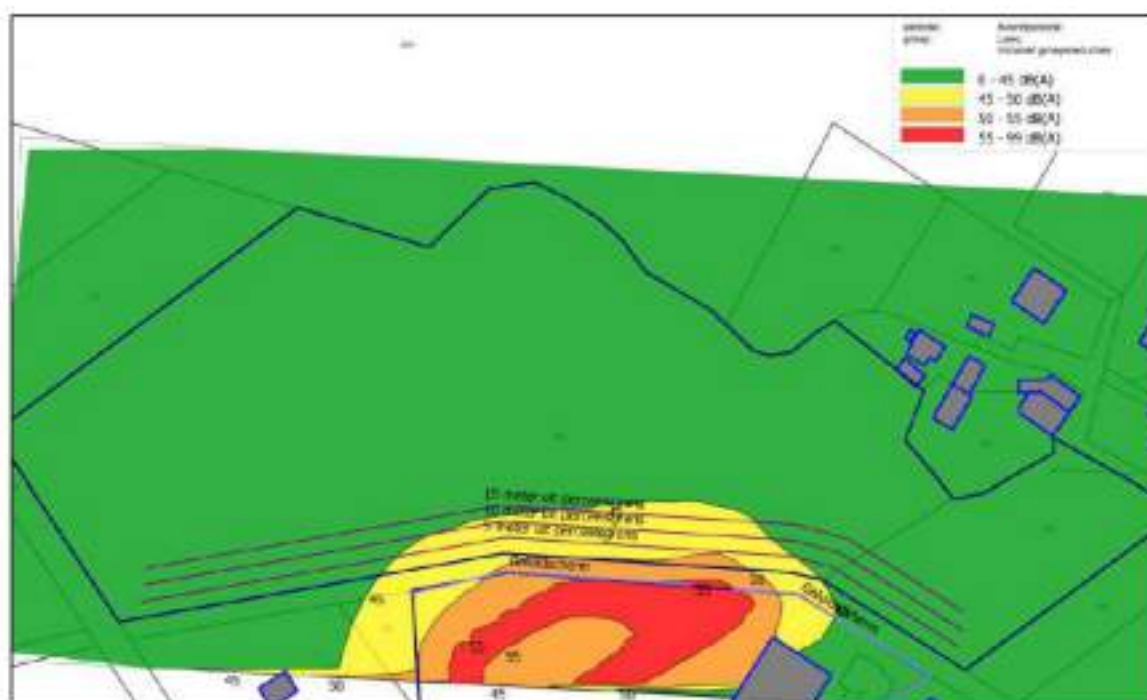
Figuur 7. Geluidscontouren op 5,0 meter in de avondperiode inclusief maatregelen
