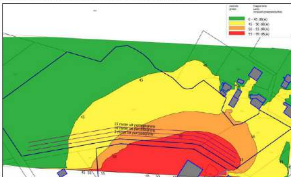
Figuur 4. Geluidscontouren plangebied woonwijk "Elzenberg" op 1,5 meter in de dagperiode
