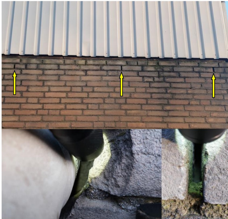
Figuur 4.4.2. De achtergevel bevat meerdere open stootvoegen (boven). Links- en rechtsonder resp. een spleet langs een pijp en een open stootvoeg.
