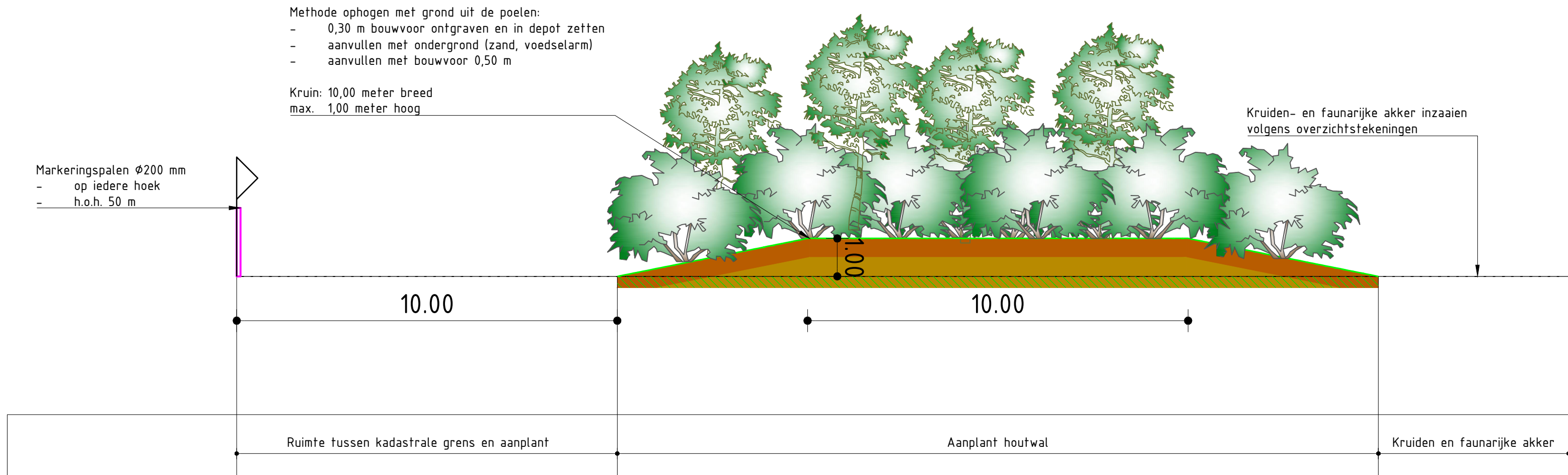
Dwarsprofiel D-D'
