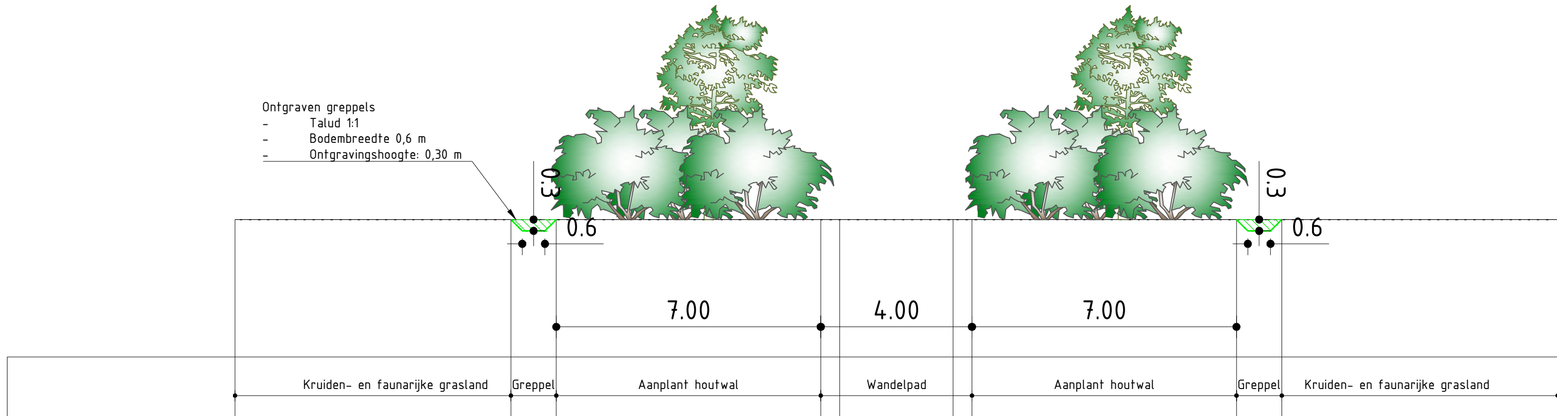
Dwarsprofiel F-F'
