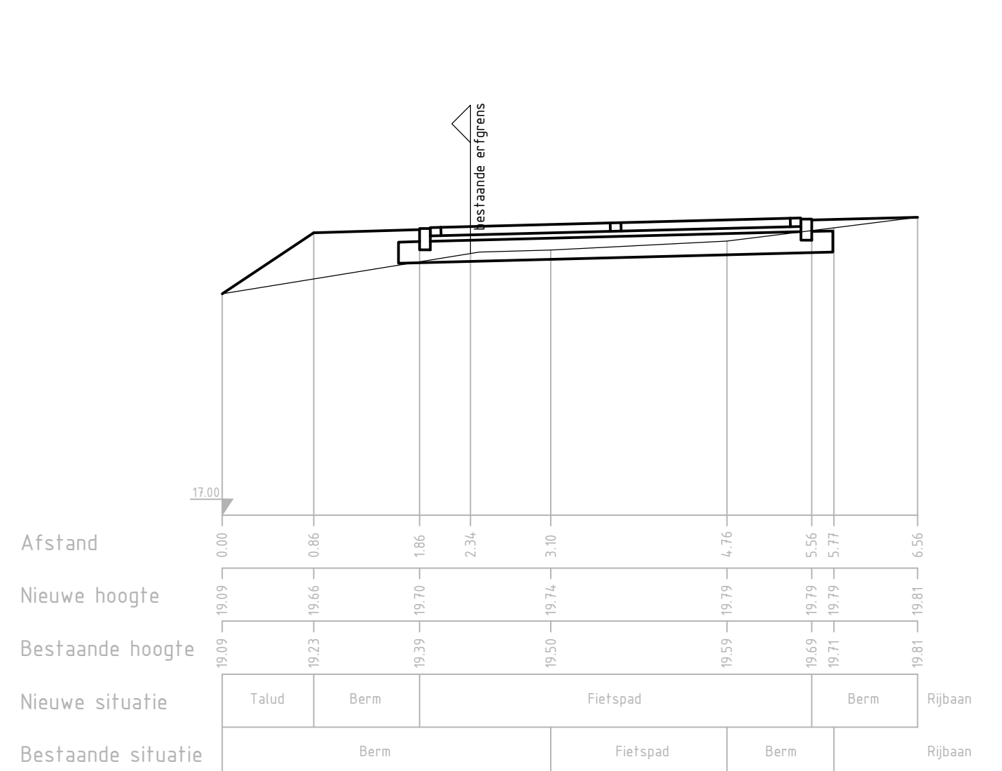
DOORSNEDE SCHAAL 1 : 50 W30 S1 Ten behoeve van: Parceel BFD20 F 1908 Eigenaar Verstraeten
