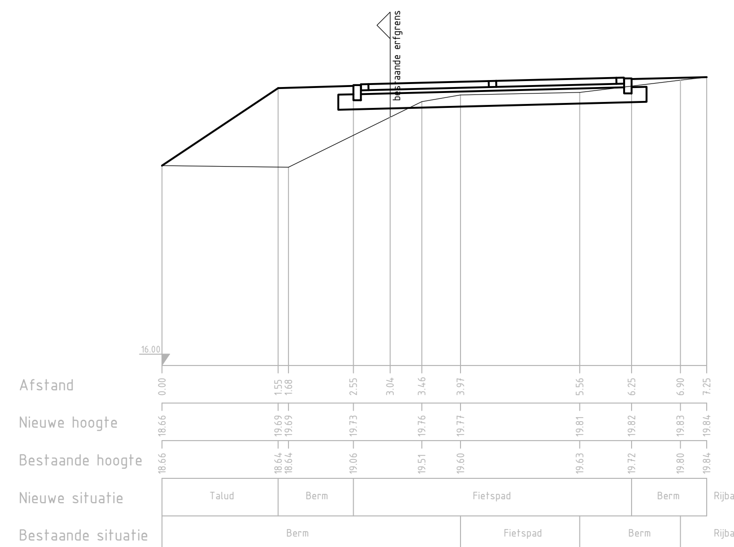
DOORSNEDE W29 Ten behoeve van: SCHAAL 1 : 50 S1 Perceel BFD00 F 1939 Eigenaar Engelen
