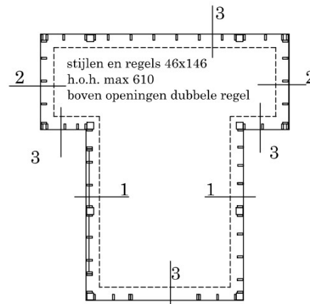
overzicht wanden
