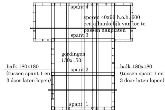
Dak
