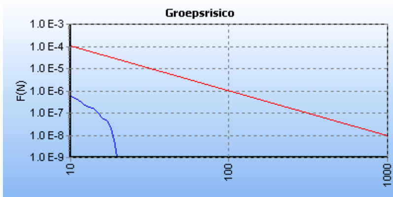
5.2 Figuur 5.2 FN curve voor Z-513-22 van N.V. Nederlandse Gasunie voor de kilometer tussen stationing 0.00 en stationing 1000.00
