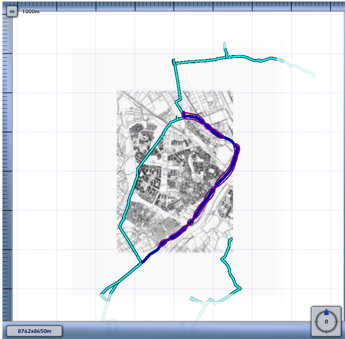
3.2 Figuur 3.2 Plaatsgebonden risico voor Z-513-22 van N.V. Nederlandse Gasunie
