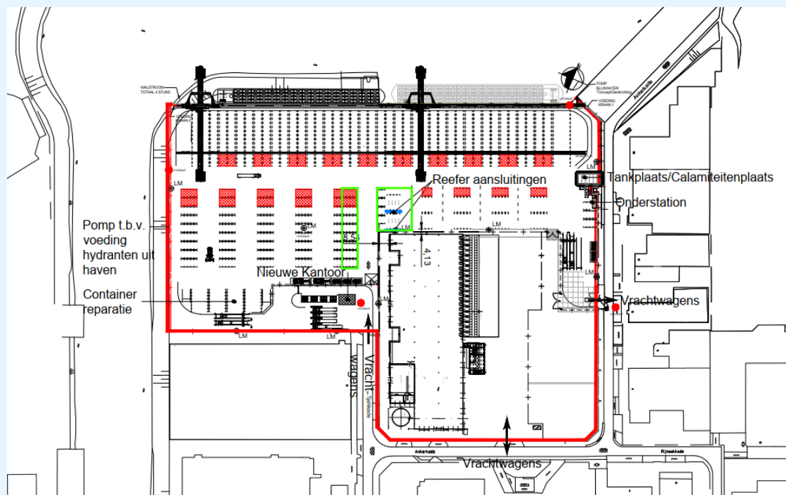
Figuur 1: inrichtingstekening van de Venlo Trade Port B.V. na de uitbreiding
