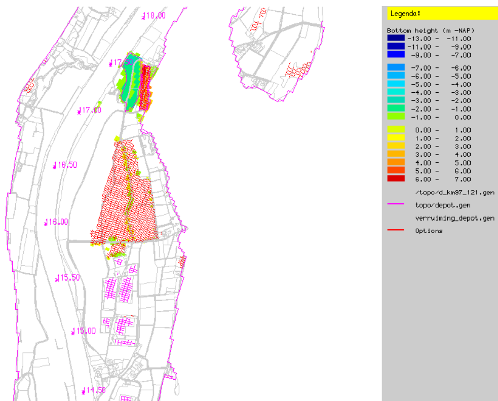
Figuur 4-5 Bodemhoogteverschil depot bypass t.o.v. vergunde situatie (rkm 114,5 – 118,5)
