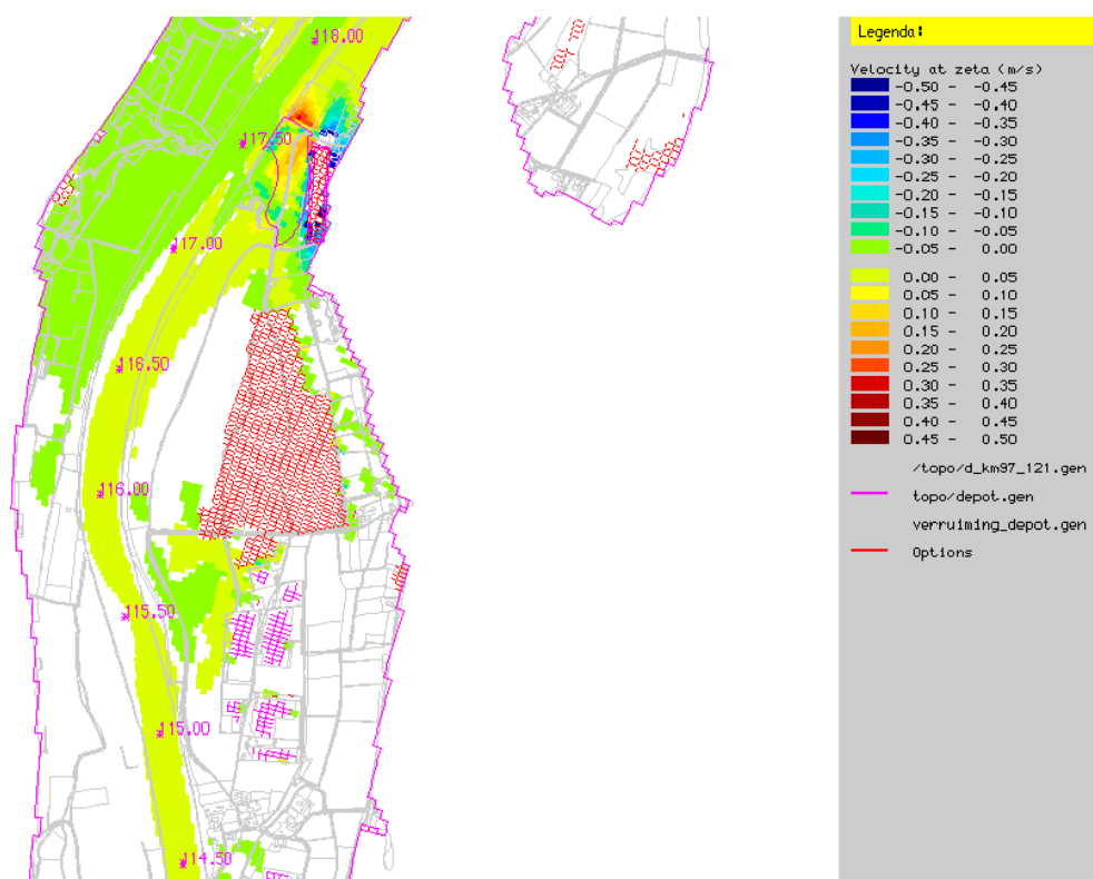
Figuur 4-11 Stroomsnelheidverschil depot bypass t.o.v. vergunde situatie, 1/1250
