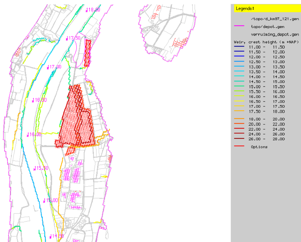
Figuur 4-4 Overlaten (ligging + hoogte) depot bypass in WAQUA-model (rkm 114,5 – 118,5)
