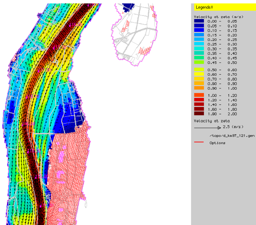
Figuur 2-5 Stroomsnelheden in de Maas (rkm 114,5 – 118,5), 1/250 Referentiesituatie
