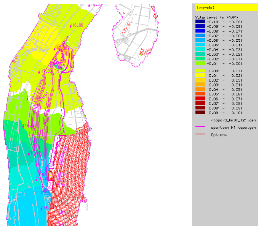
Figuur 3-8 Waterstandverschil BPRW-ontwerp t.o.v. Referentiesituatie, 1/250
