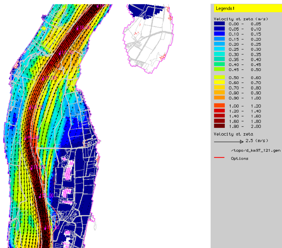
Figuur 2-8 Stroomsnelheden in de Maas (rkm 114,5 – 118,5), 1/1250 Referentiesituatie
