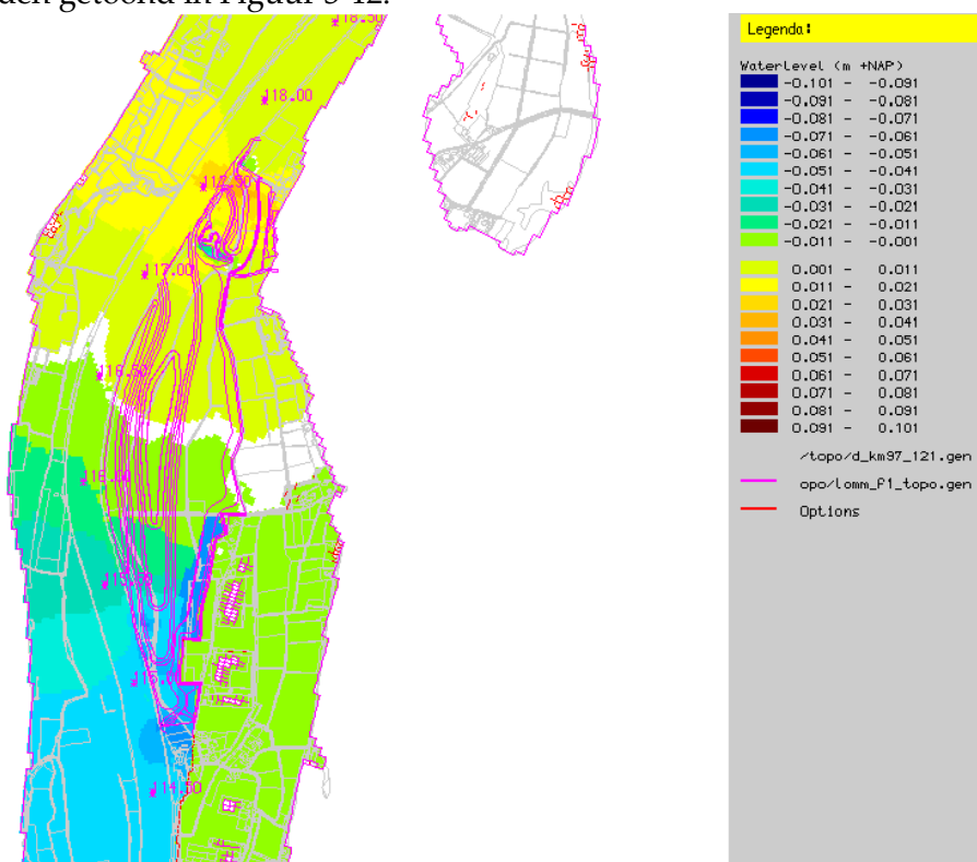
Figuur 3-11 Waterstandverschil BPRW-ontwerp t.o.v. Referentiesituatie, 1/1250
