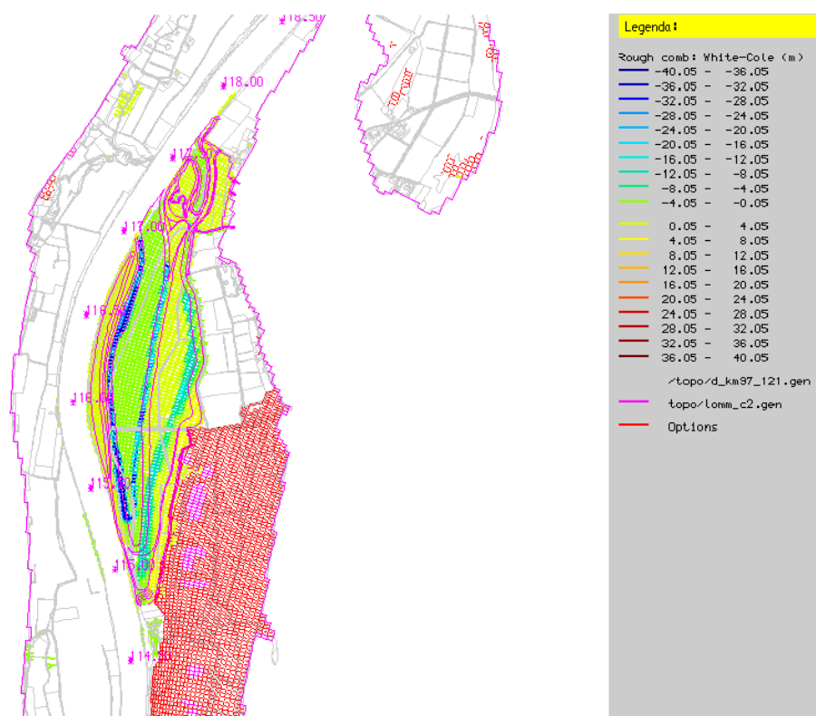
Figuur 4-12 Ruwheidverschil (m) Alternatief 2 t.o.v. Nulalternatief (rkm 114,5 – 118,5)
