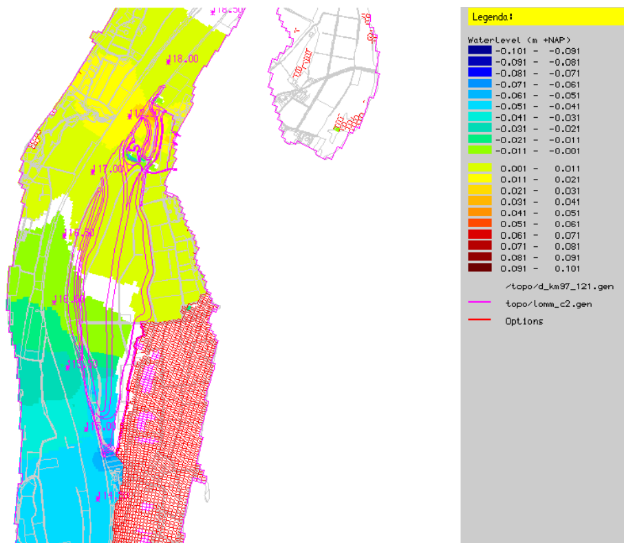
Figuur 4-13 Waterstandverschil (m), Alternatief 2 t.o.v. Nulalternatief, 1/250 situatie
