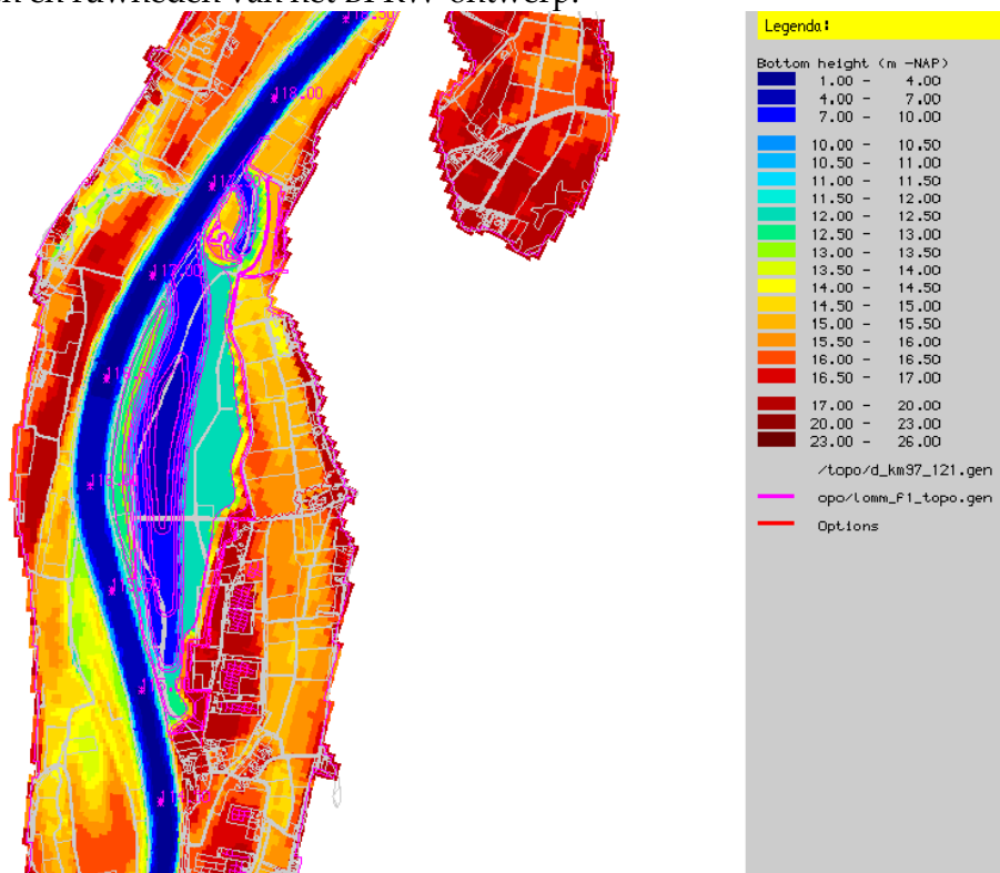
Figuur 3-3 Bodemhoogte BPRW-ontwerp in WAQUA-model (rkm 114,5 – 118,5)
