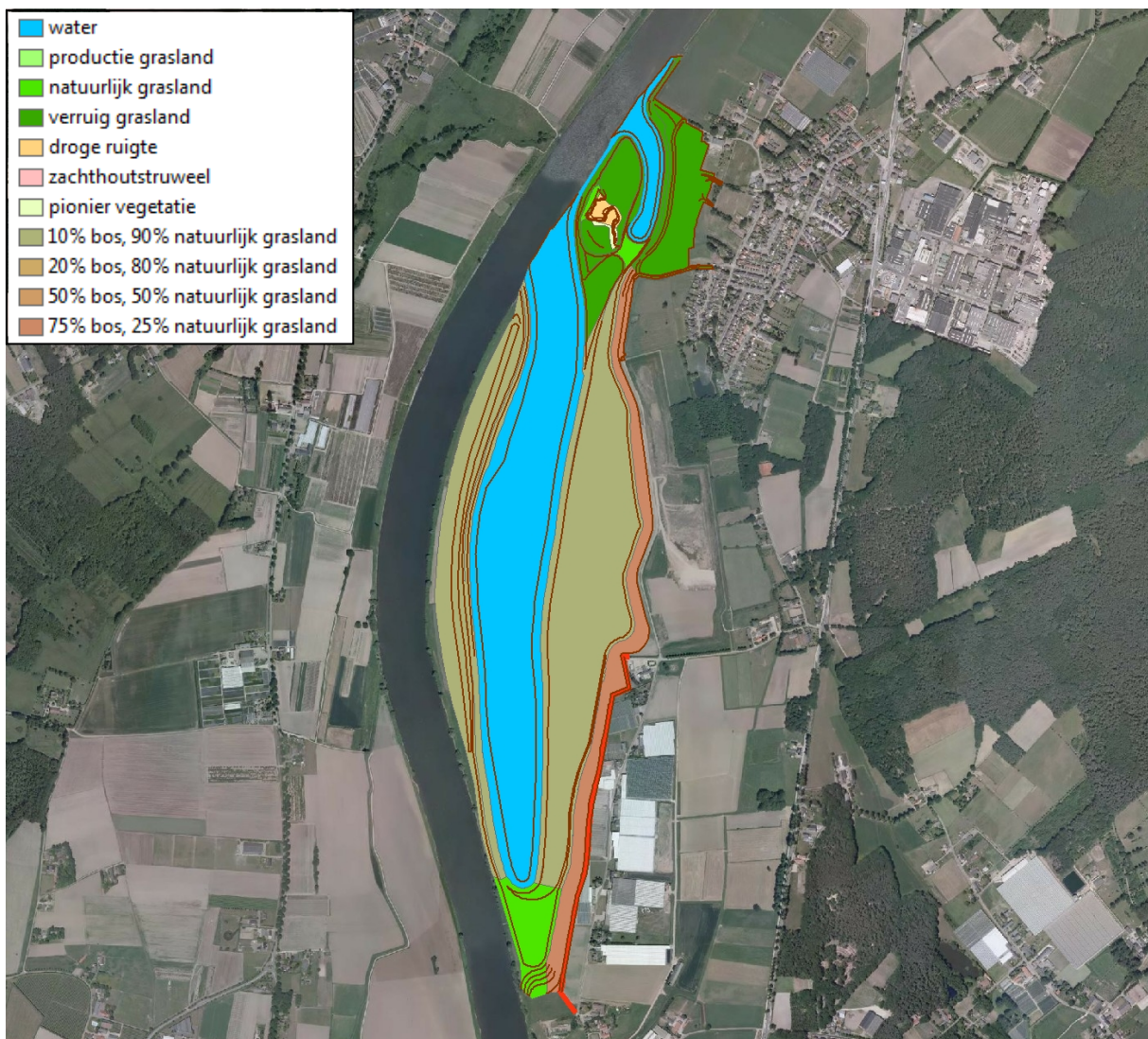
Figuur 4-2 Inrichtingsplan Alternatief 1 hoogwatergeul Lomm
