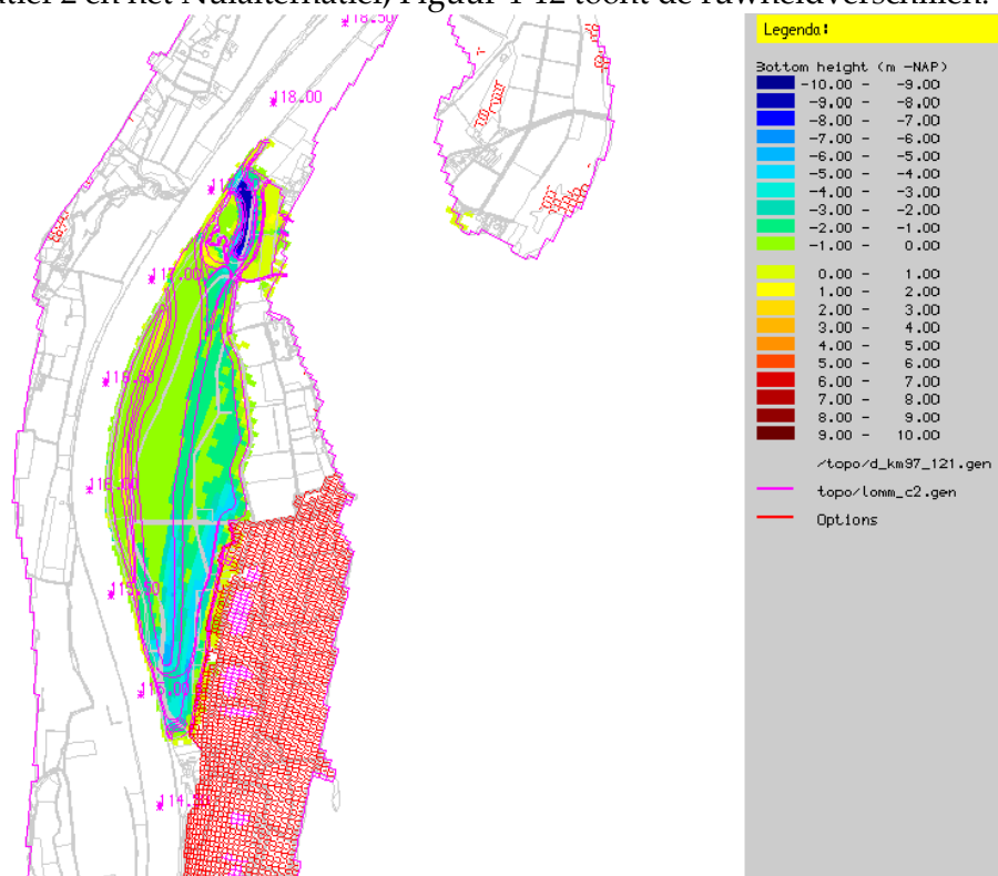
Figuur 4-11 Bodemhoogteverschil (m) Alternatief 2 t.o.v. Nulalternatief (rkm 114,5 – 118,5)
