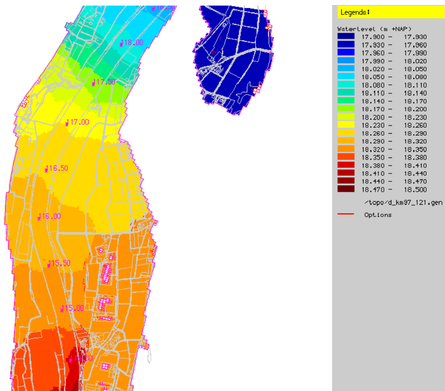
Figuur 2-6 Waterstanden in de Maas (rkm 114,5 – 118,5), 1/1250 Referentiesituatie
