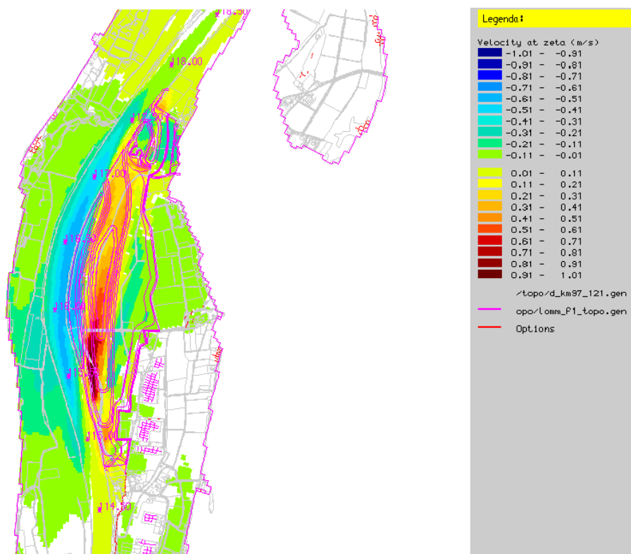
Figuur 3-13 Stroomsnelheidverschil BPRW-ontwerp t.o.v. Referentiesituatie, 1/1250
