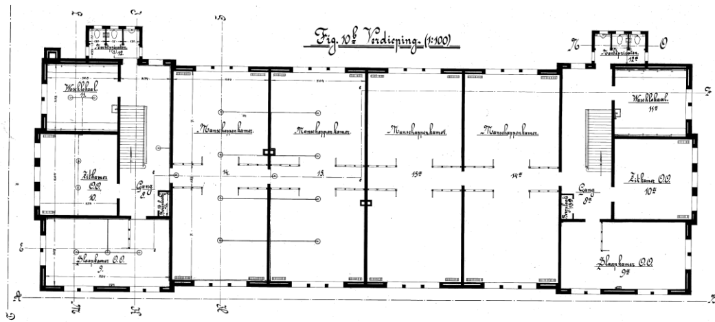
Figuur 30 Bouwtekening
