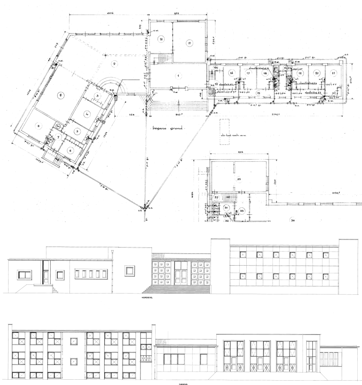
Figuur 51 Bouwtekeningen gebouw J
