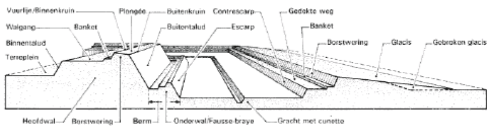
DWARSPROFIEL 1/6 VESTINGWAL
