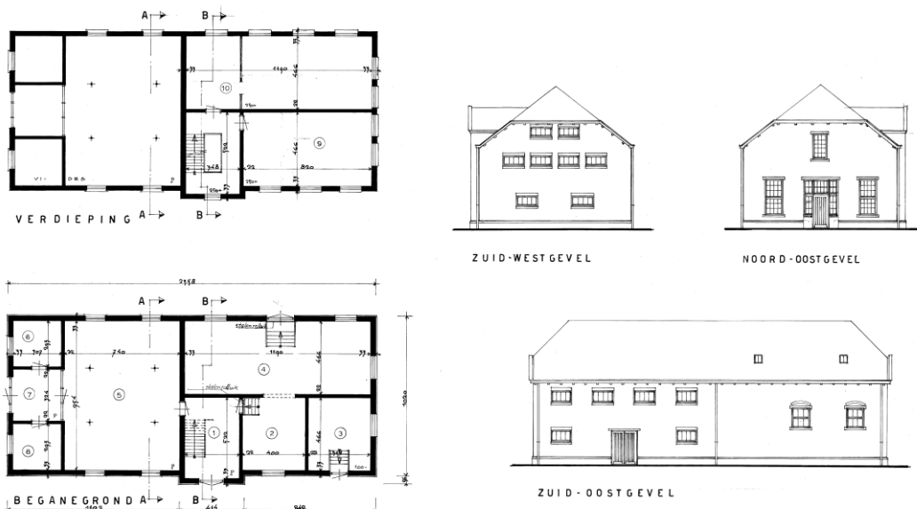
Figuur 33 Bouwtekeningen
