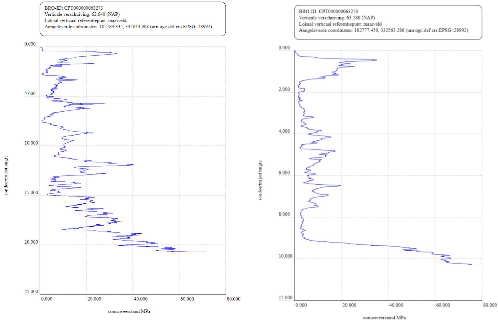
Figuur 1: BODEMWEERSTAND AFGELEID VAN SONDERINGEN IN DE OMGEVING VAN HET ONDERZOEKSGBIED. BRON: DINOLOKET.
