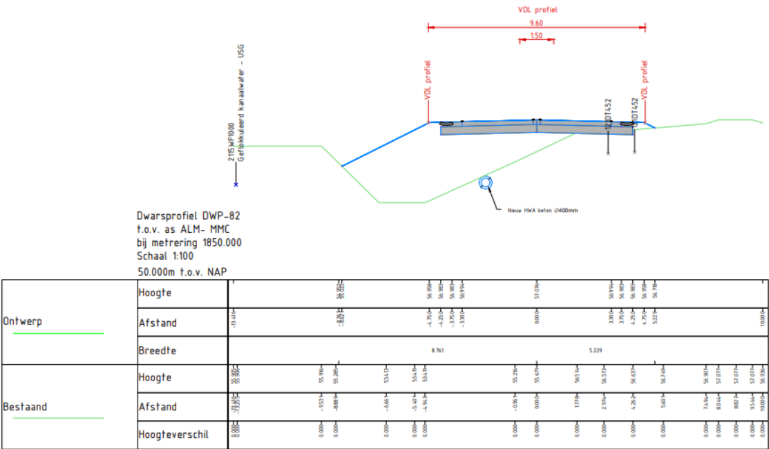
Figuur 19. Dwarsprofiel DWP-82 ter hoogte van het grote waterbekken in Sittard-Geleen.
