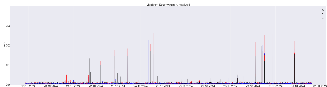
figuur 6 Trillingsniveaus locatie meetpunt Spoorweglaan (Orion03)
