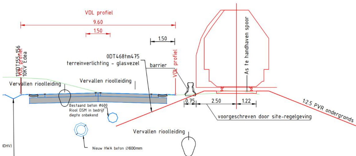
Figuur 2: doorsnede ligging weg en spoor
