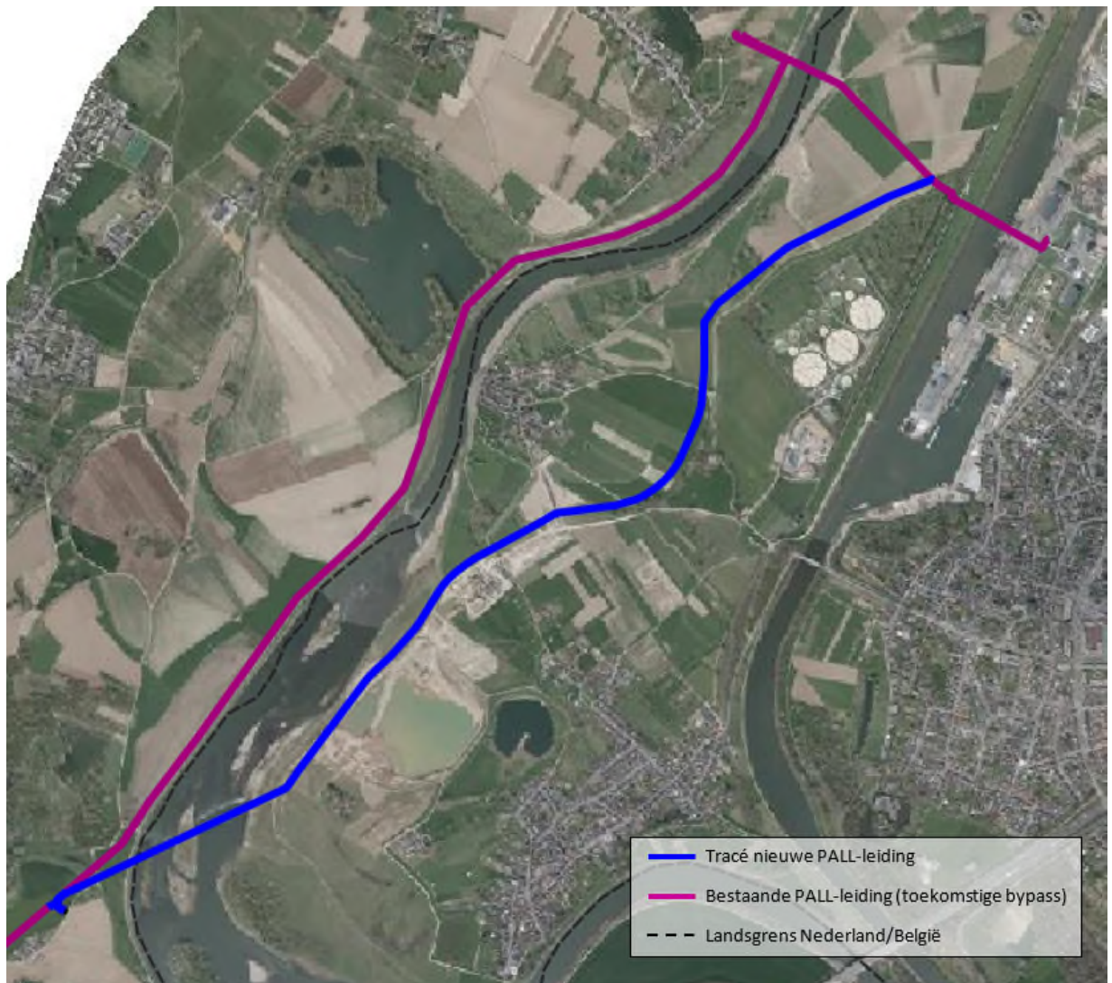
Figuur 2.1 Indicatieve ligging nieuwe PALL-leiding
