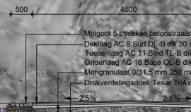
Normaalprofiel D-D Schaal 1:50
