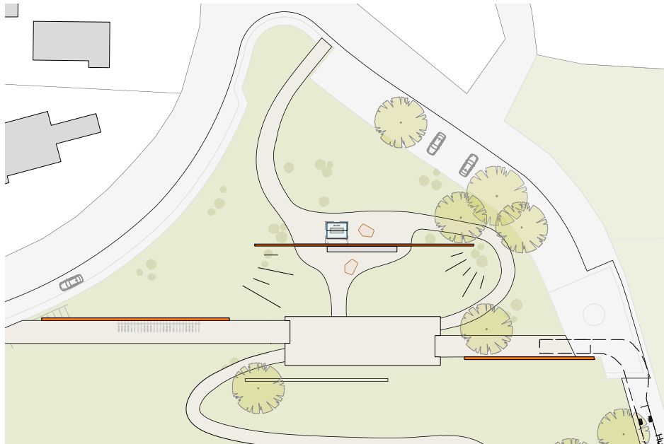
LANDSCHAP: Landschappelijk plan met keerwanden en uitzichtpunt, "balkon"
