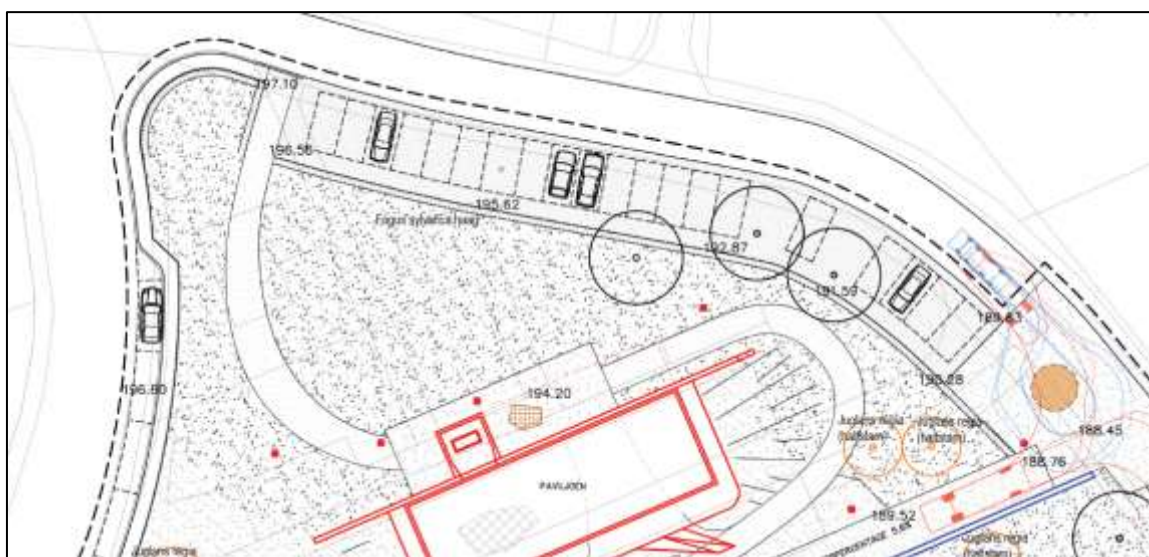
Parkeren noordzijde via Hulsbergweg
