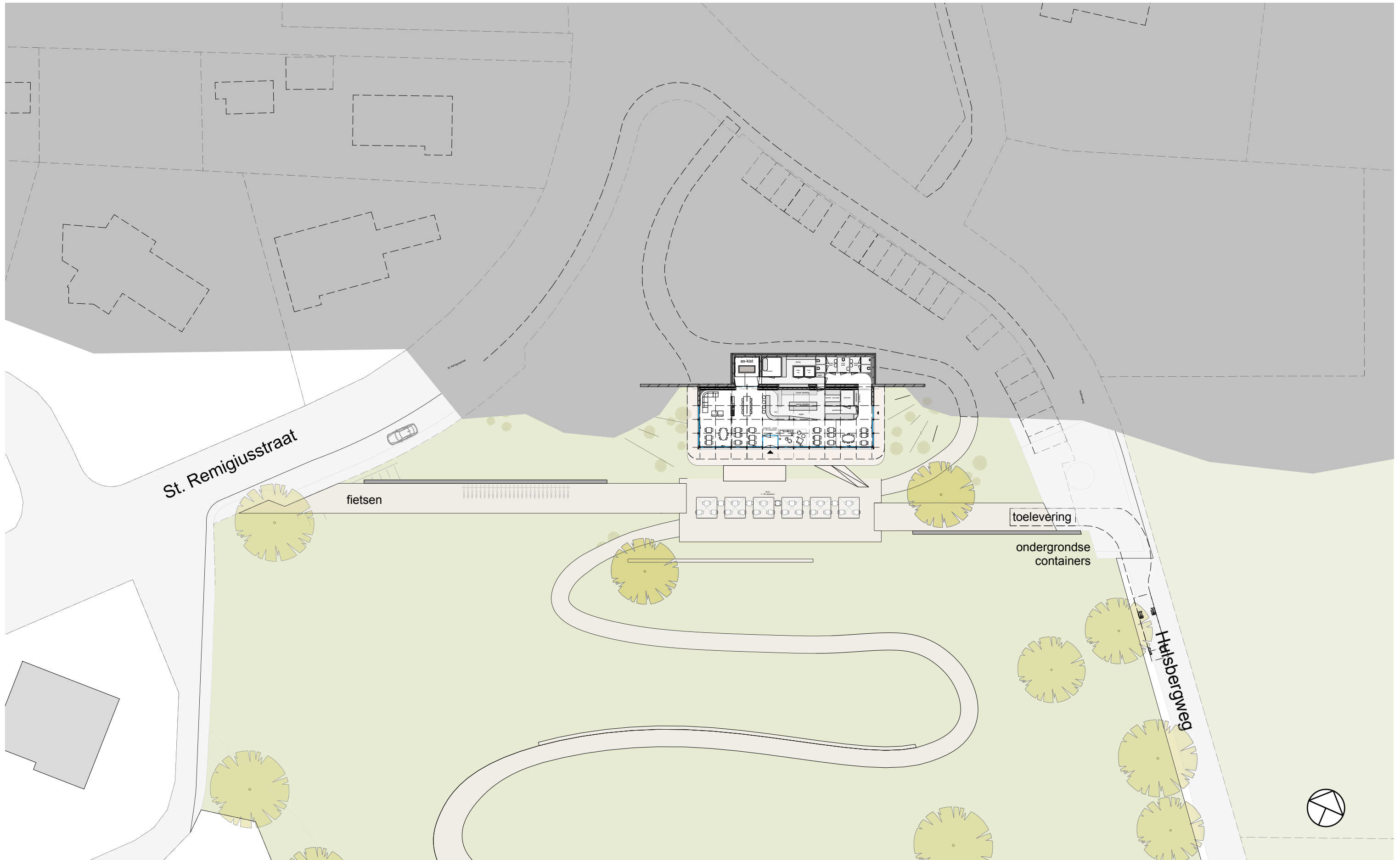
plattegrond | 1:500
