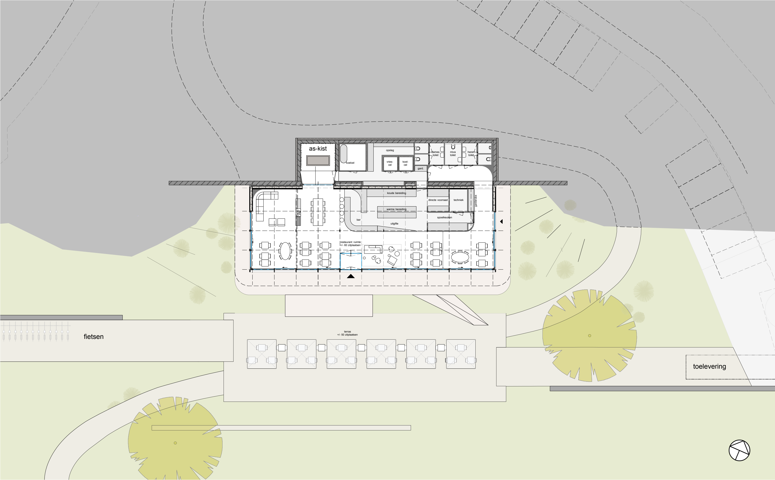
plattegrond | 1:200
