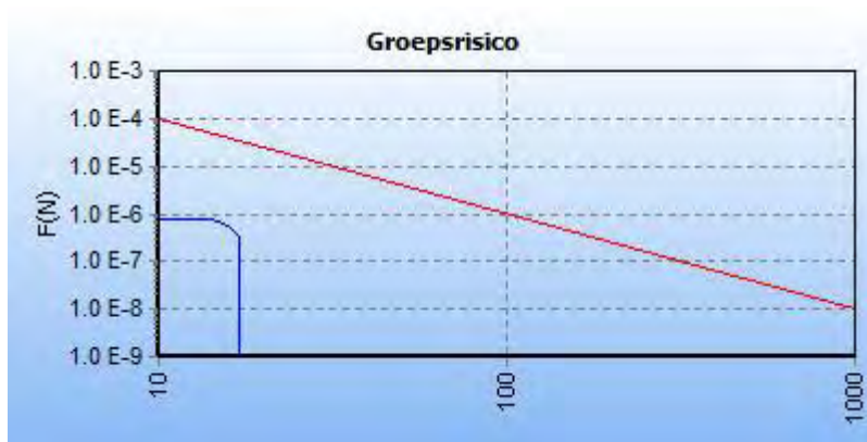
5.1 Figuur 5.1 FN curve voor 7549_leiding-Z-509-05-deel-1 van N.V. Nederlandse Gasunie voor de kilometer tussen stationing 630.00 en stationing 1630.00
