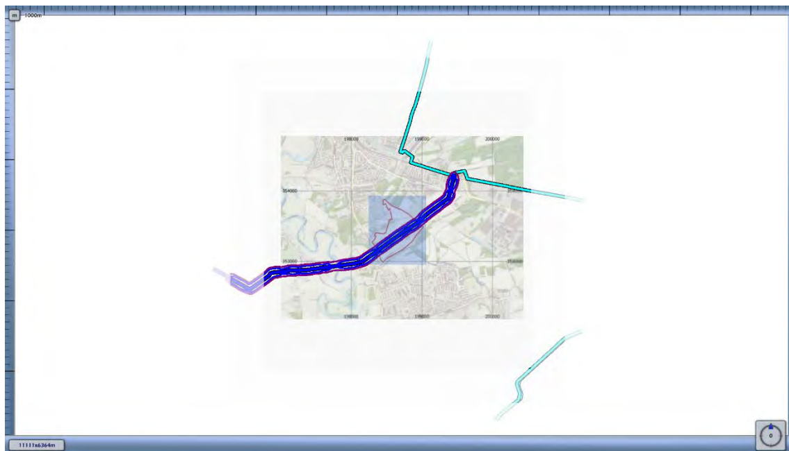
3.1 Figuur 3.1 Plaatsgebonden risico voor 7549_leiding-Z-509-05-deel-1 van N.V. Nederlandse Gasunie
