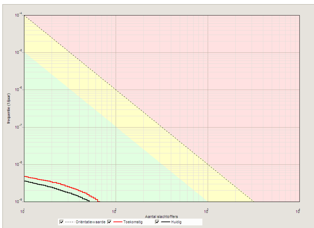
Figuur 5. Groepsrisicocurven A73
