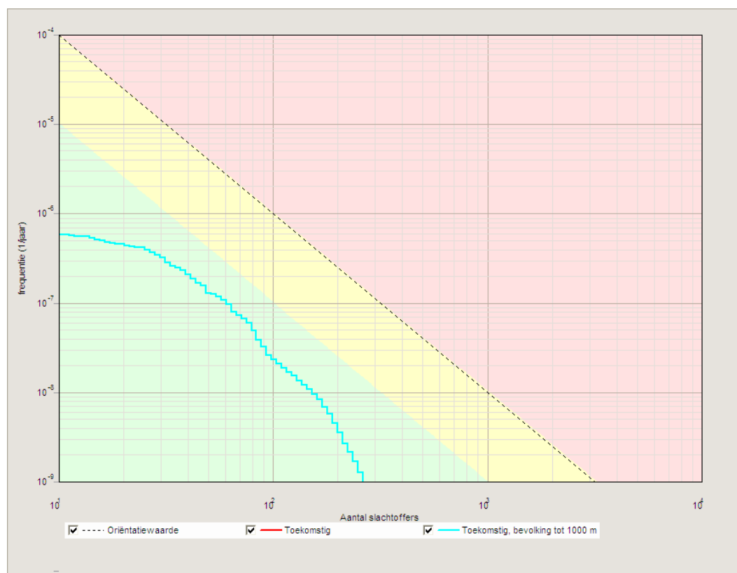
Figuur 10. GR-curven bevolking tot 300 m en tot 1000 m vanaf de weg
