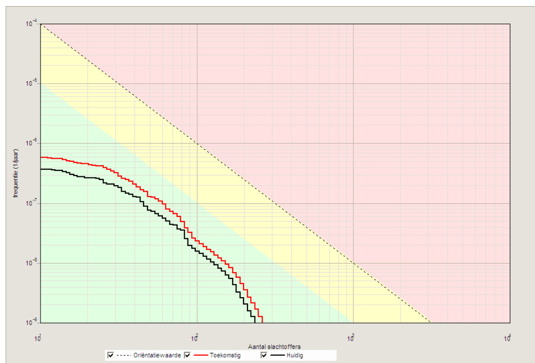
Figuur 3. Groepsrisicocurven A73
