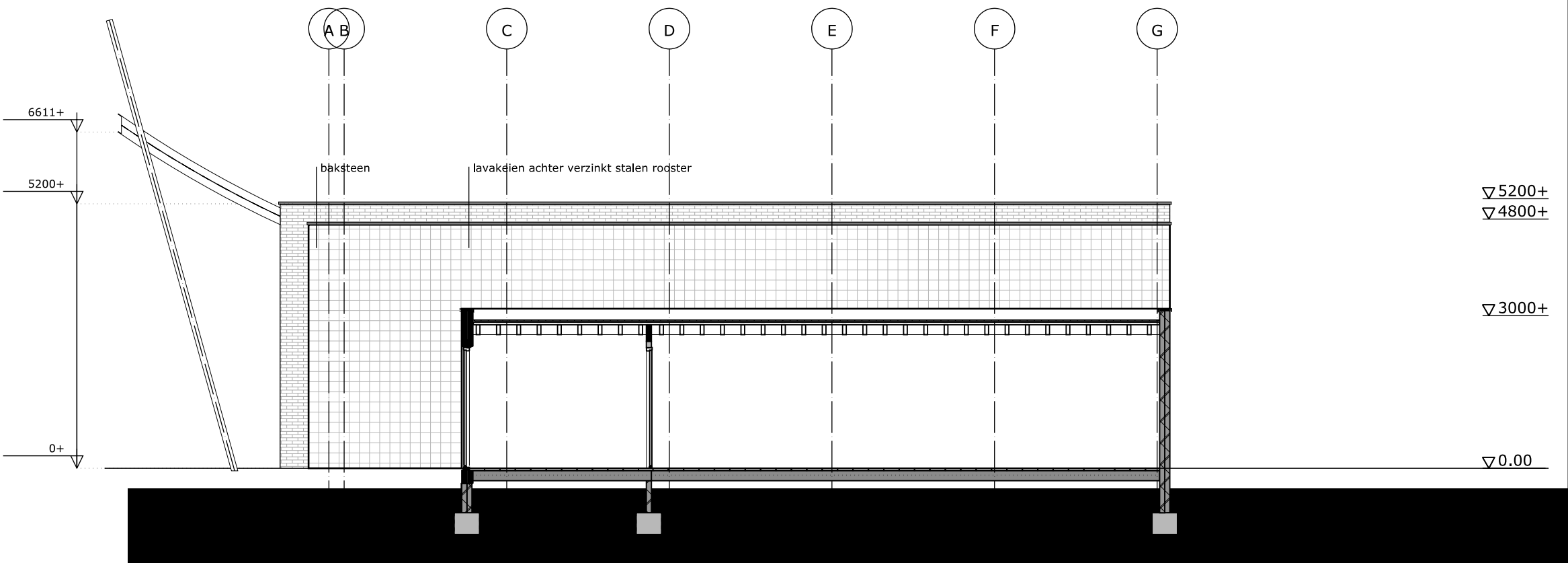
rechter zijgevel
