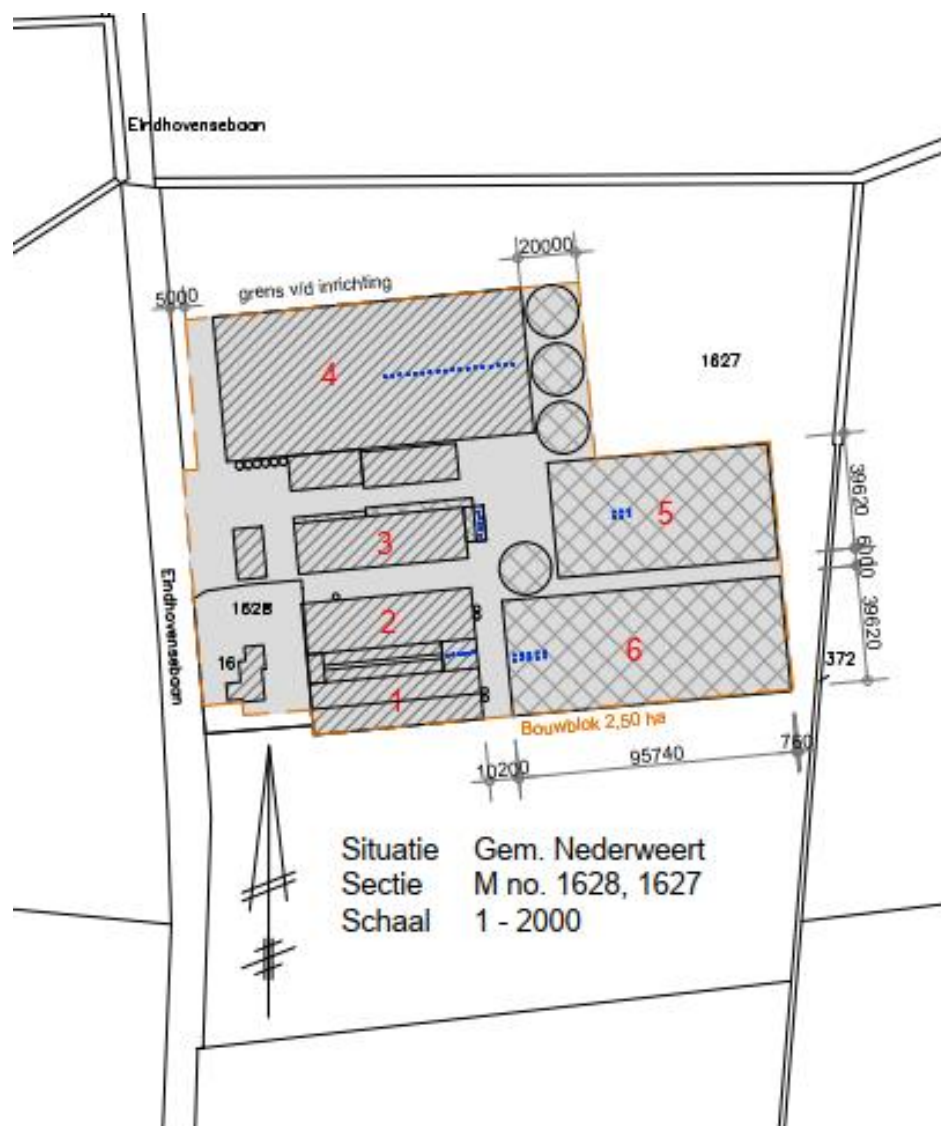
Situatieschets voornemen door uitbreiding stal 5 en 6
