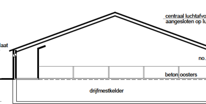
- Doorsnede C - C gebouw 2 -
