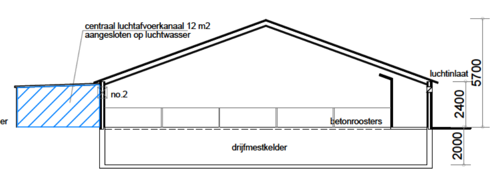
- Doorsnede D - D gebouw 1 -
