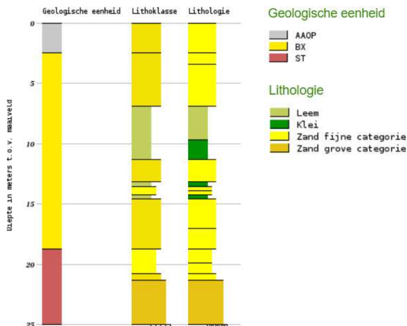
Figuur 9: Bodemprofiel t.h.v. de Brugstraat (bron: Dinoloket).
