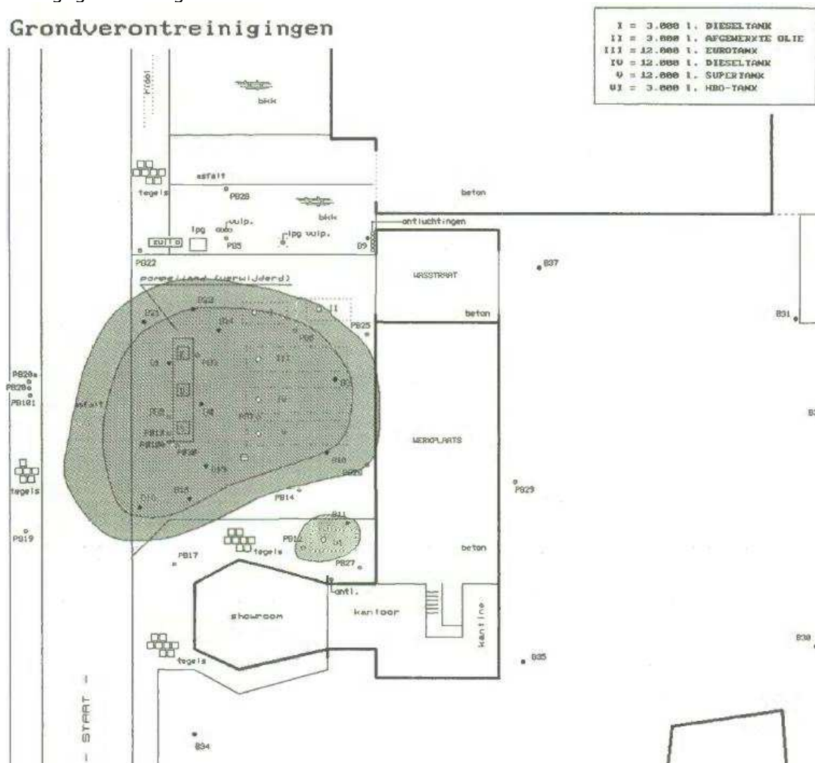
Figuur 5: Tekening voormalige verontreinigingscontour binnen Staat 42
