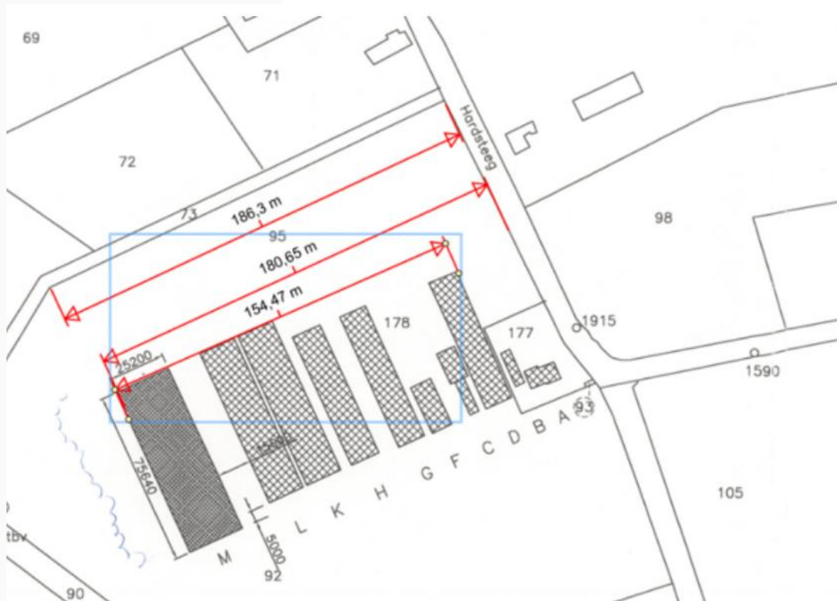
Figuur 1.3.1.2 Uitsnede situatietekening BV 2004029
