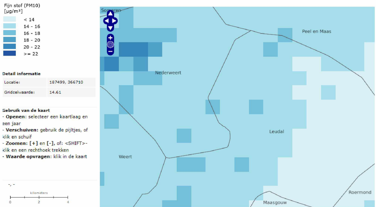
Figuur 4-2 Concentratie PM 10 in de omgeving van het plangebied (GCN 2023)
