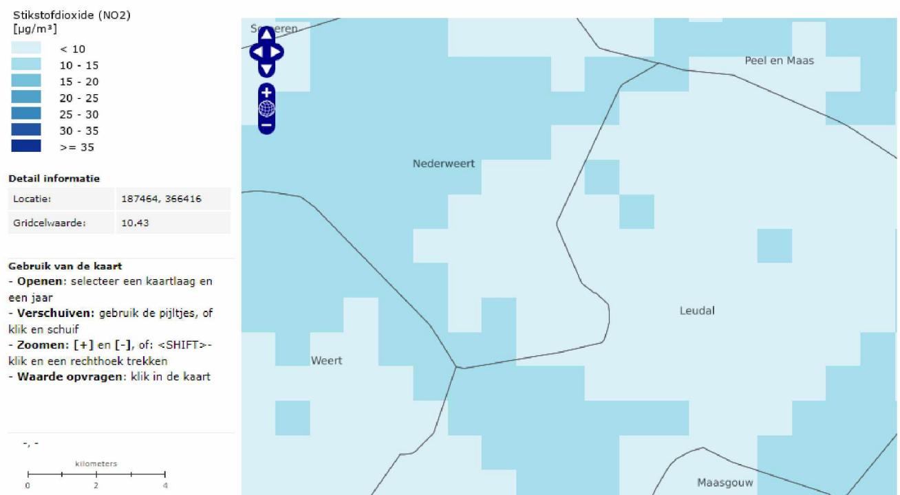
Figuur 4-1 Concentratie \text{NO}_2 in de omgeving van het plangebied (GCN 2023)
