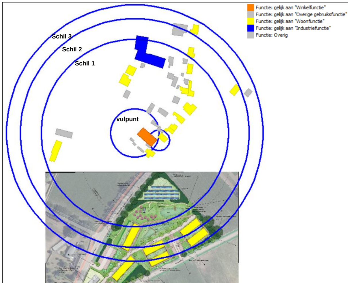
Figuur 4.2 Invloedsgebied rondom vulpunt (toekomstige situatie)
