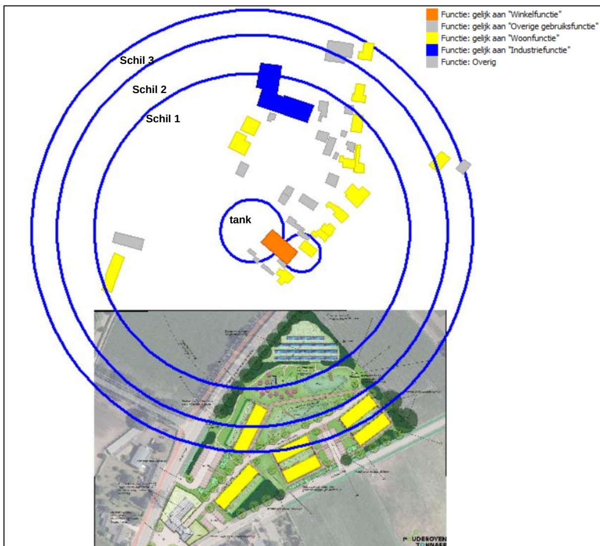
Figuur 4.1 Invloedsgebied rondom ingeterpte tank (toekomstige situatie)
