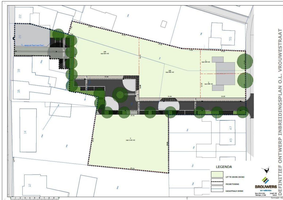
Figuur 9. Definitief ontwerp O.L. Vrouwestraat te Ospel (bron: Adviesbureau Brouwers).
