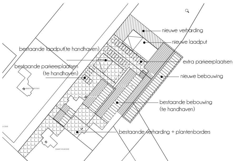
Situatie parkeerplaatsen (bestaand en uitbreiding)
