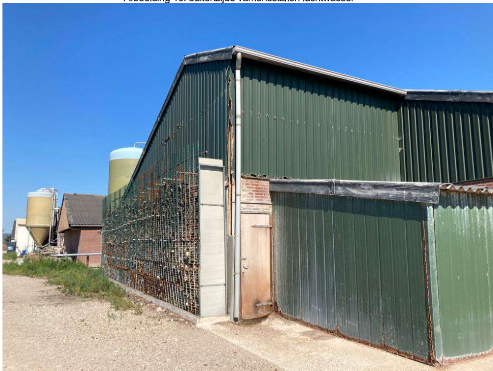
• Afbeelding 10: buitenzijde varkensstallen luchtwasser
