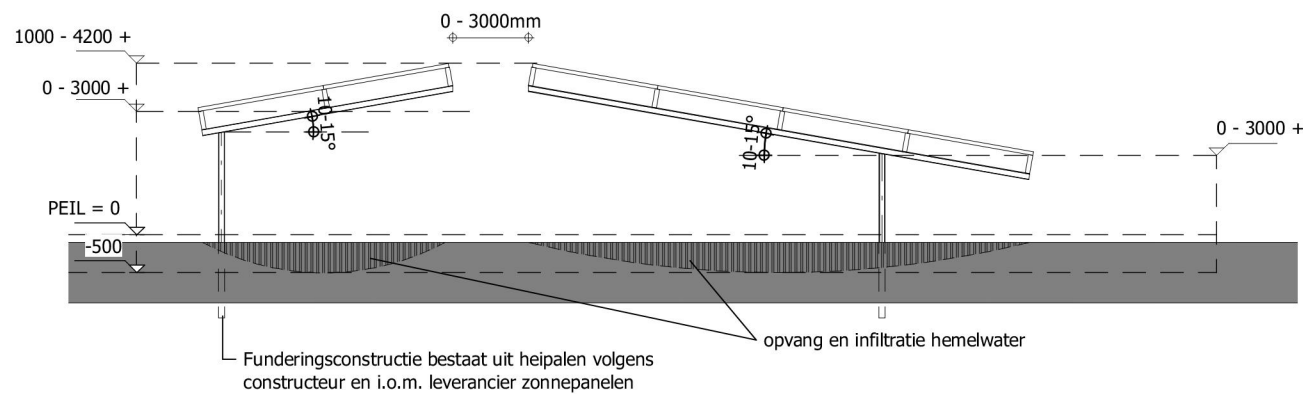
ACHTERAANZICHT ZONNEPANELEN
