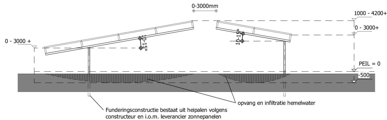
VOORAANZICHT ZONNEPANELEN
