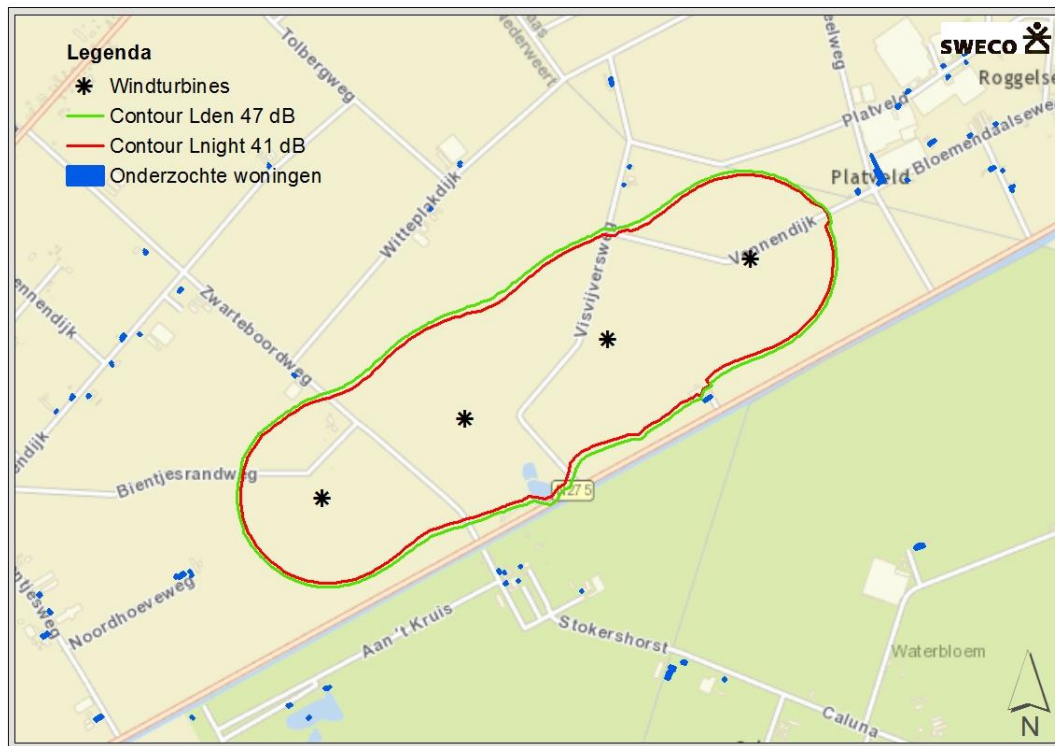
Figuur 3.1 Geluidscontouren onder Activiteitenbesluit 47 dB L_{den} en 41 dB L_{night}
