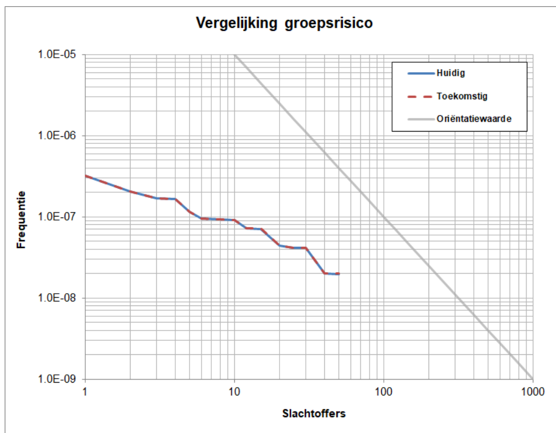
Figuur 3. Groepsrisicovergelijking bij doorzet tot 1500 m 3 /jr
