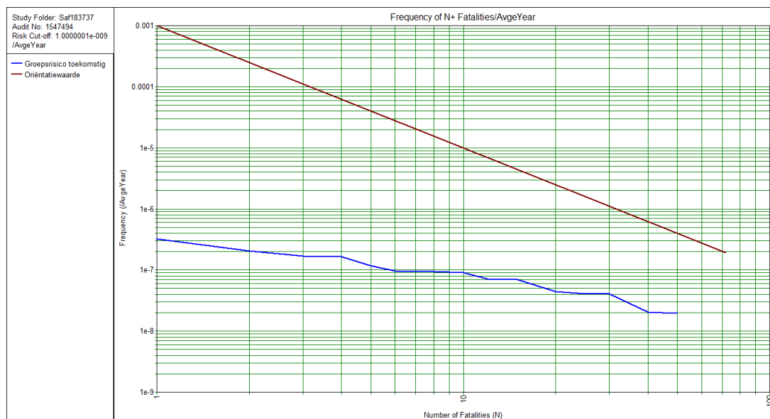
Figuur 5. Groepsrisico toekomstige situatie met doorzet tot 1500 m³/jr
