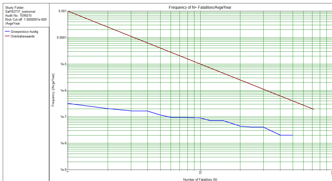
Figuur 4. Groepsrisico huidige situatie met doorzet tot 1500 m³/jr
