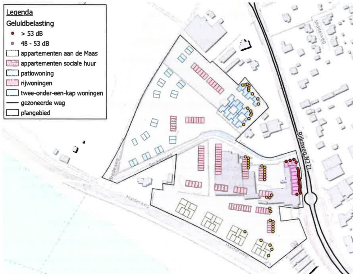
Figuur 1: Toetspunten met een overschrijding van de ten hoogste toelaatbare geluidsbelasting als gevolg van verkeer op de Rijksweg N271.
