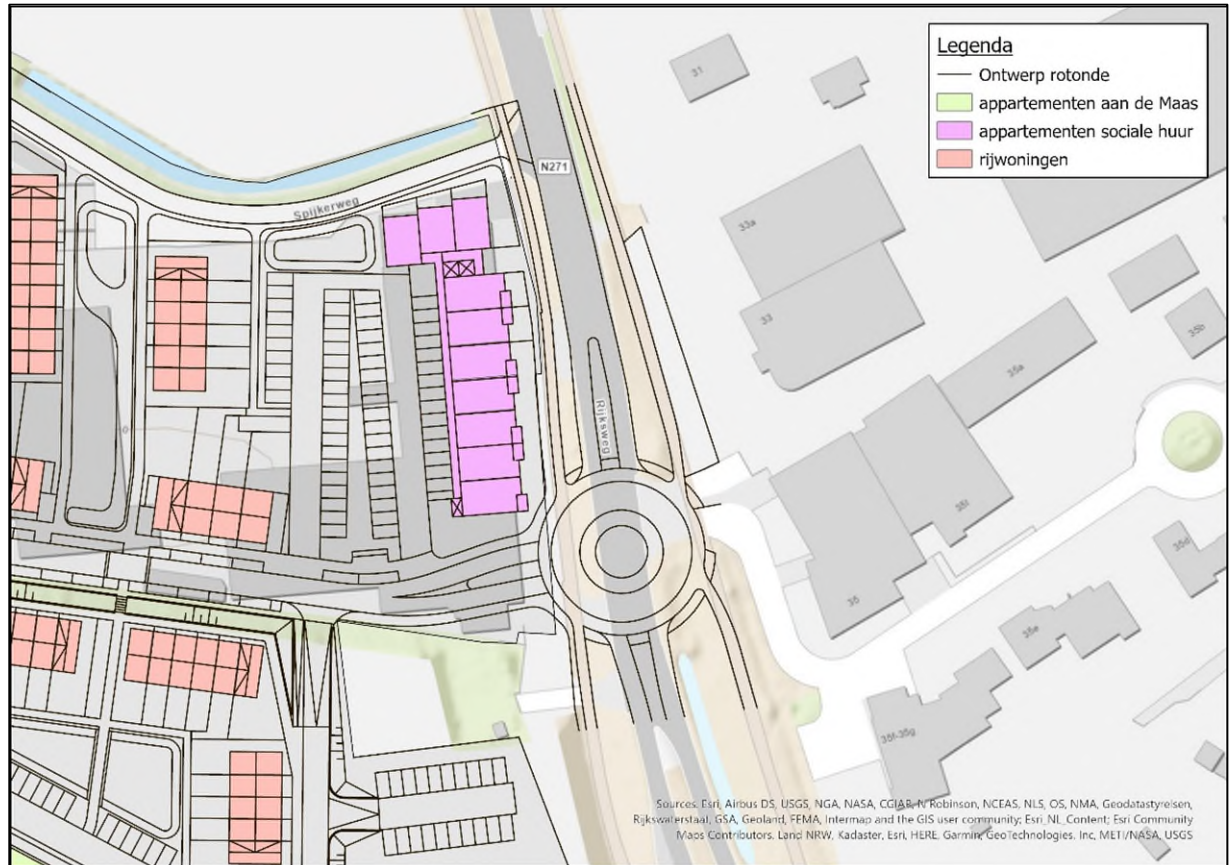
Figuur 3.2 Ontwerp van de rotonde als wijziging aan de Rijksweg N271.
