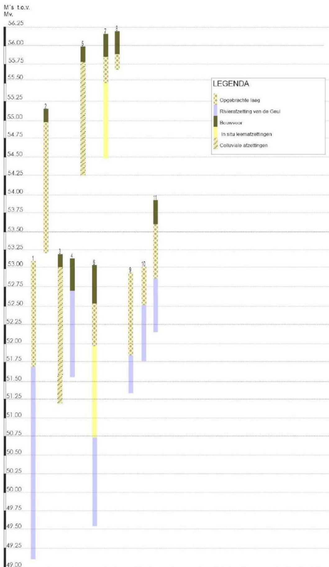
Figuur 24: Boorprofielen.
