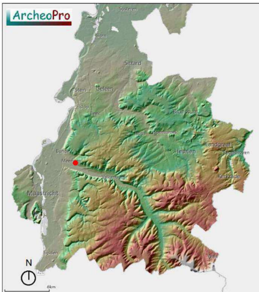
Figuur 5: Hoogtekaart van het Zuid-Limburgse lössgebied met in rood de ligging van het plangebied. 7
