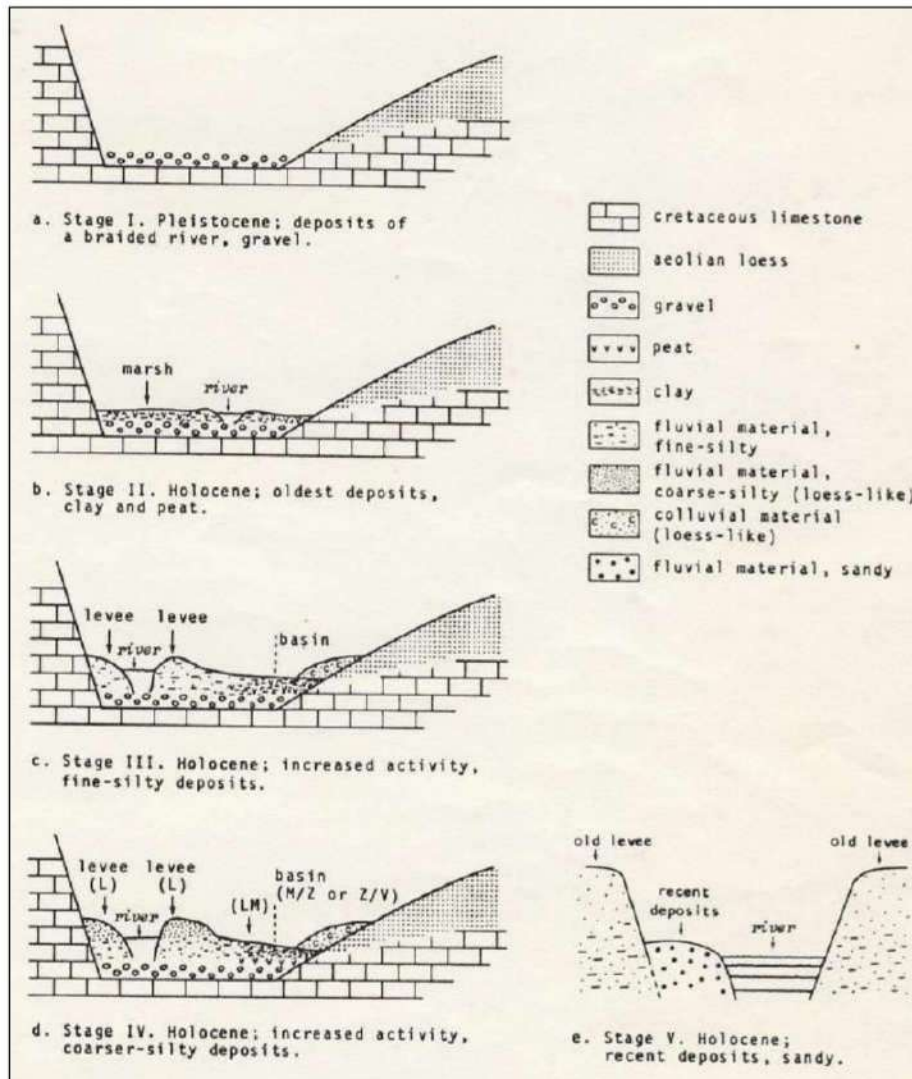
Figuur 6: Schematisch lithogenetisch dwarsprofiel van het Geuldal. 12
