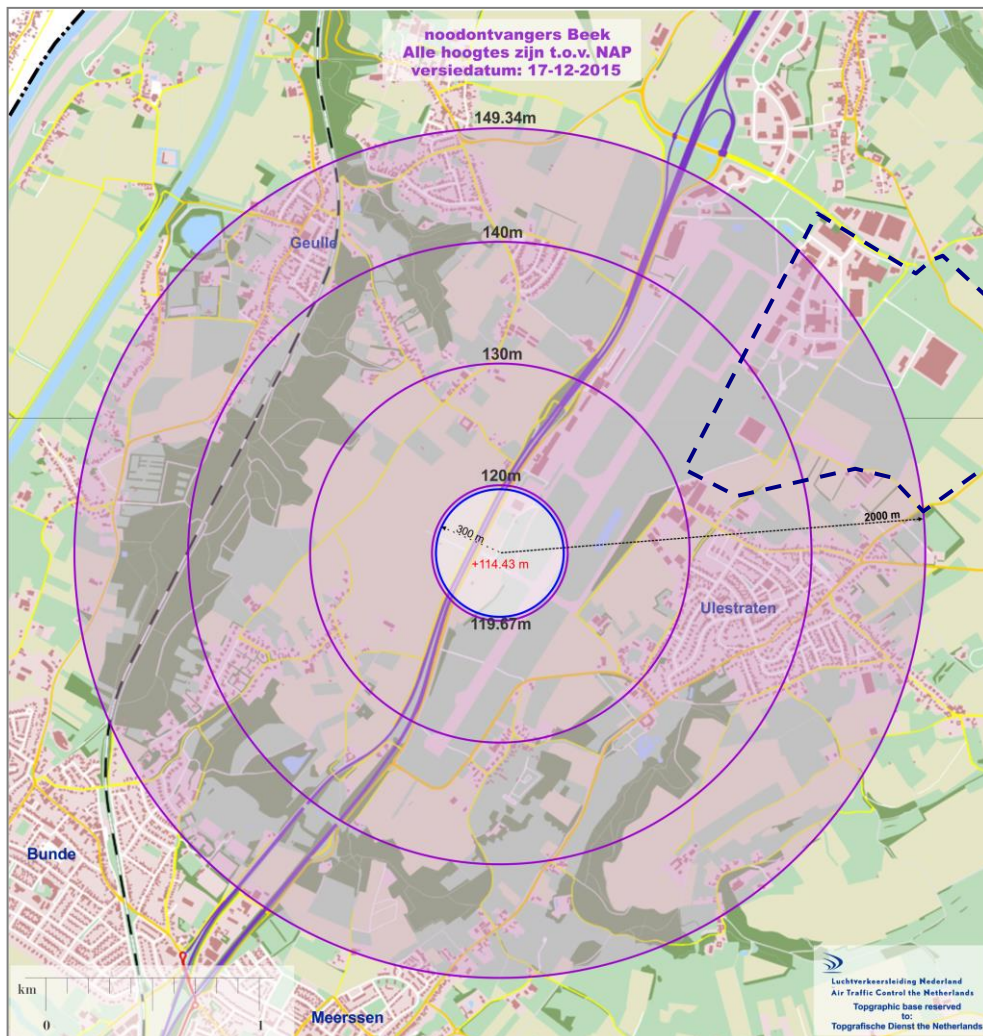
Toetsingsvlakken noodontvangers Beek (plangebied ligt binnen blauwe lijn)
