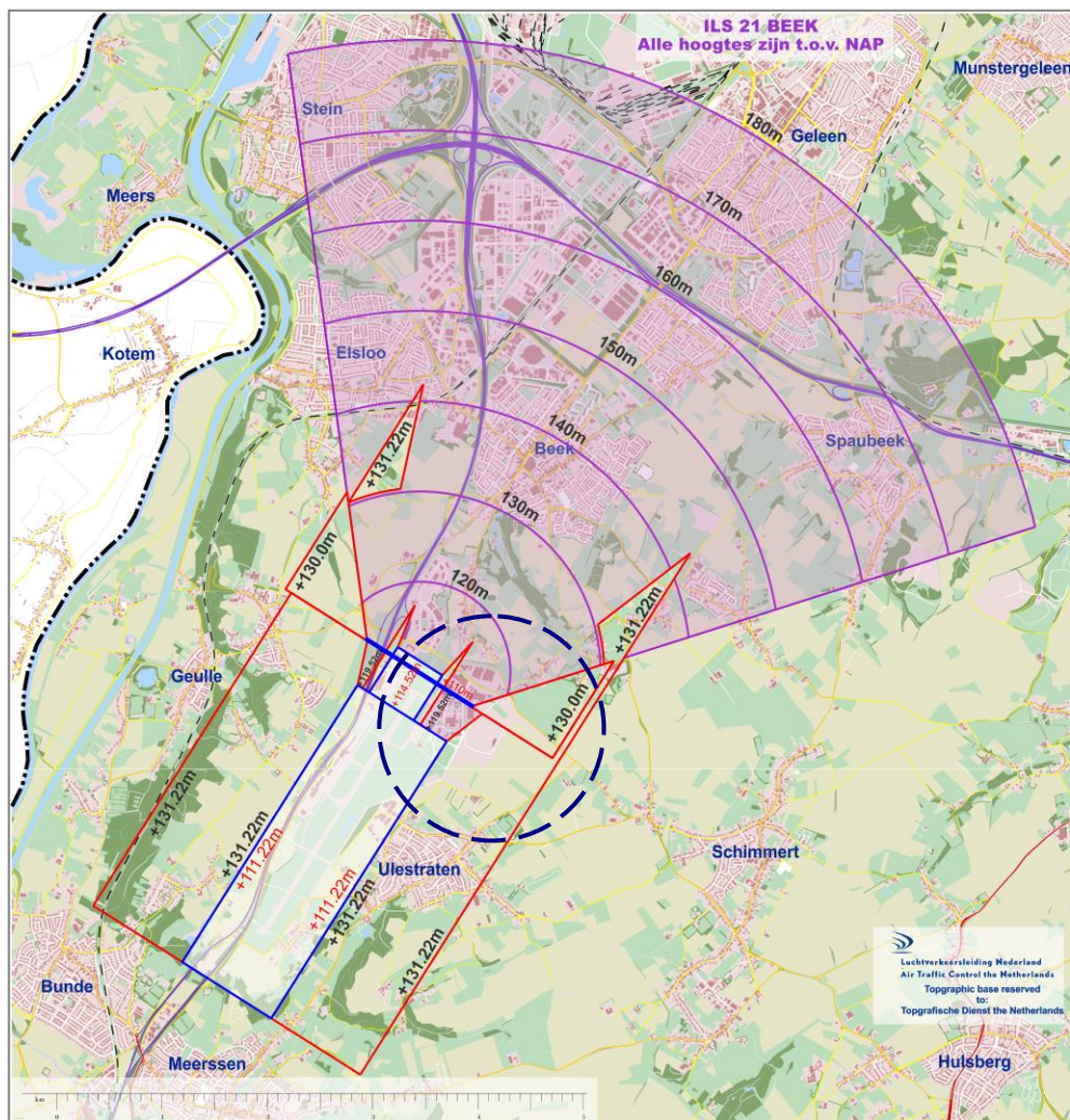
Toetsingsvlakken Instrument Landing System 21 (plangebied ligt in blauwe cirkel)
