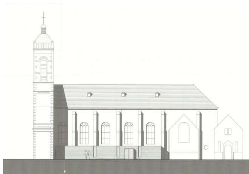
Afbeelding 31 Rechter zijgevel (zuid)
