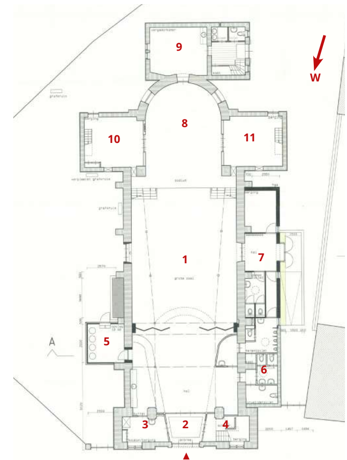
Afbeelding 27 Plattegrond Sint-Agneskerk
