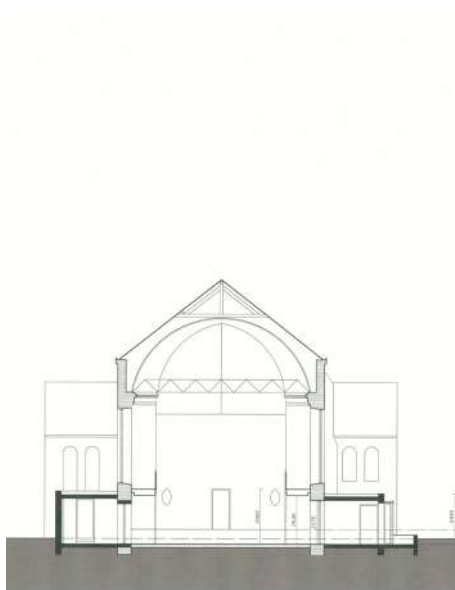
Afbeelding 30 Verticale doorsnede
