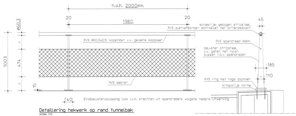
Detailing hekwerk op rand tunnelbak
