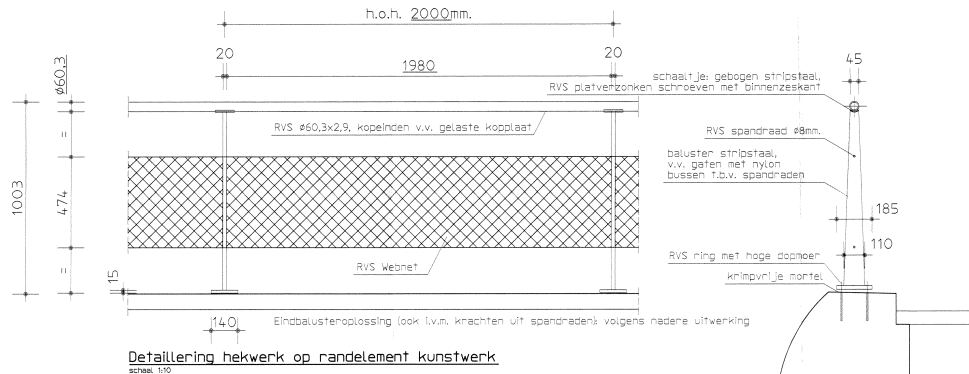
Detailing hekwerk op randelement kunstwerk
